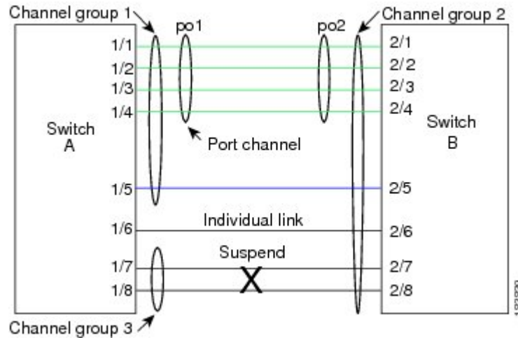
図 2: 個々のリンクをポートチャネルに組み込む
