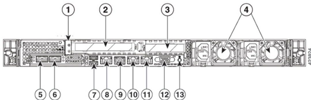
図 2: アプライアンスの背面パネル
