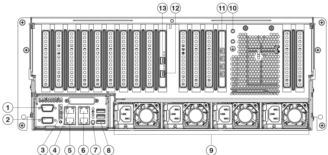
図 4: 112 コアアプライアンスの背面パネル
