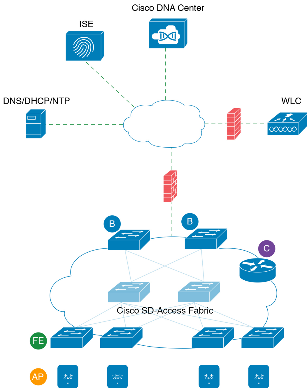
図 10 : Cisco SD-Access ファブリック インフラストラクチャ
