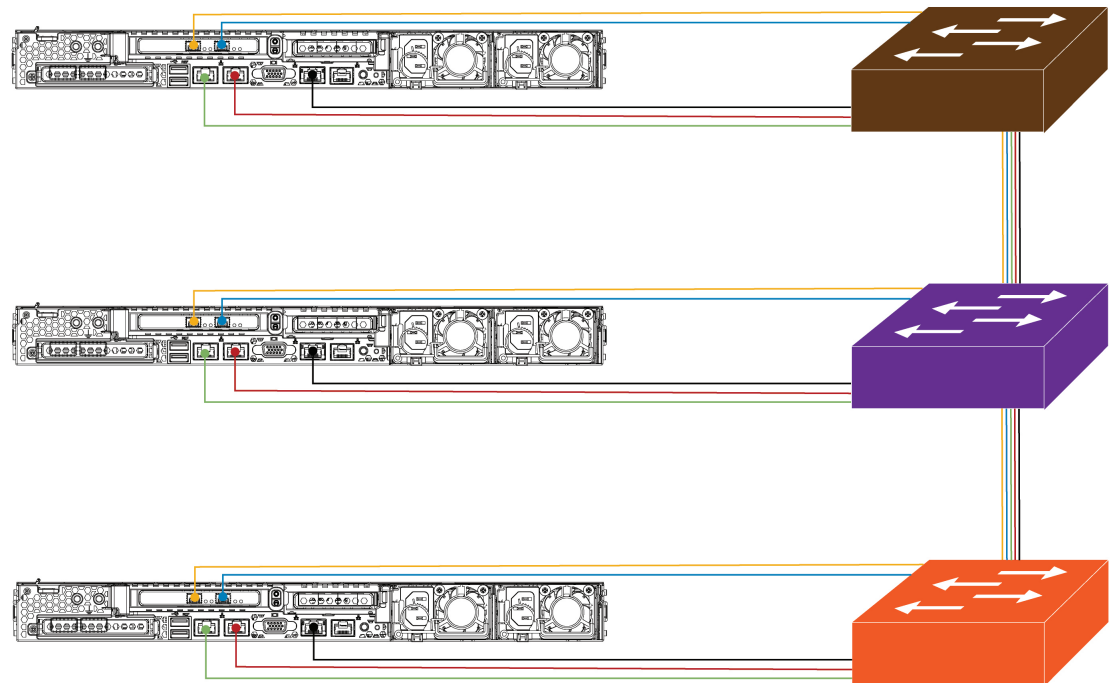
図 8:3 ノードクラスターで推奨されるケーブル接続 : 44 および 56 コアアプライアンス
