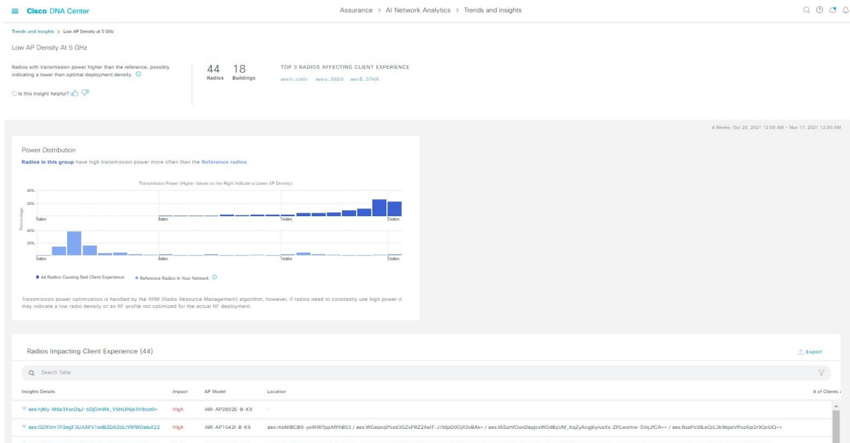
図 37: 影響を受ける無線のインサイト サマリー ダッシュボード
