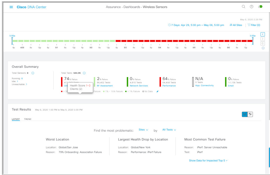
図 31 : [Wireless Sensors] ダッシュボード
