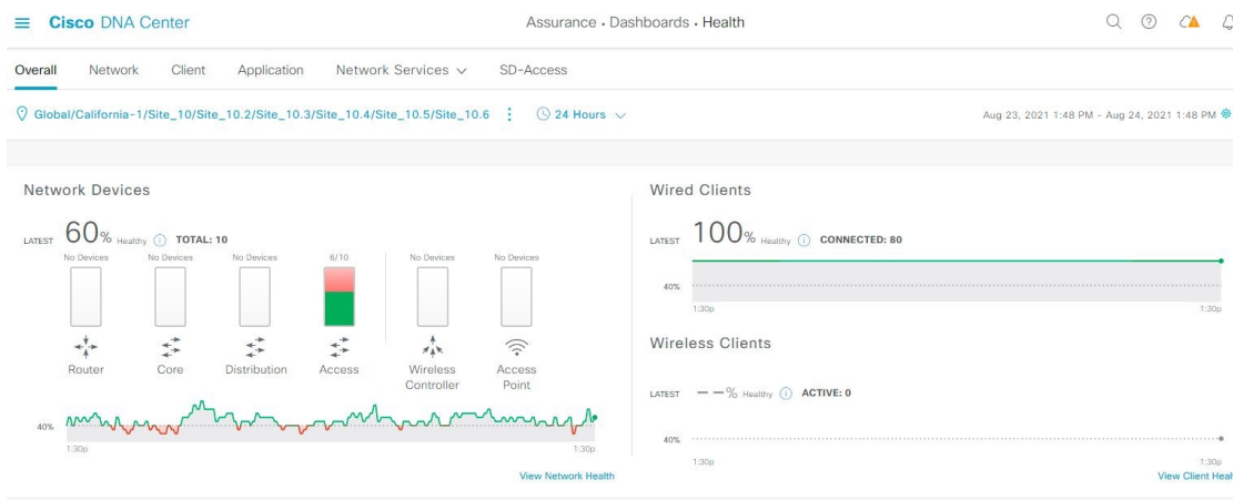
図 10 : [Overall Health] ダッシュボード
