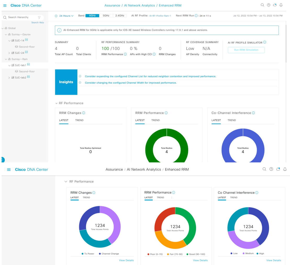
図 44: 機能強化された RRM ダッシュボード
