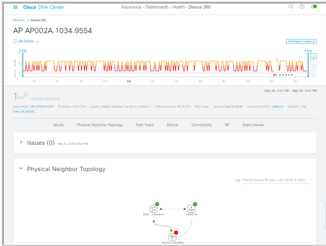
図 7: [Device 360] ウィンドウ
