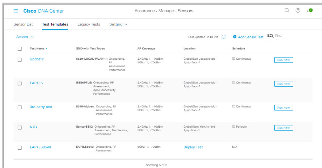
図 34: [Test Templates] ウィンドウ
