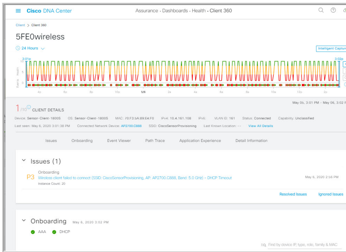
図 2: [クライアント 360 (Client 360)] ウィンドウ
