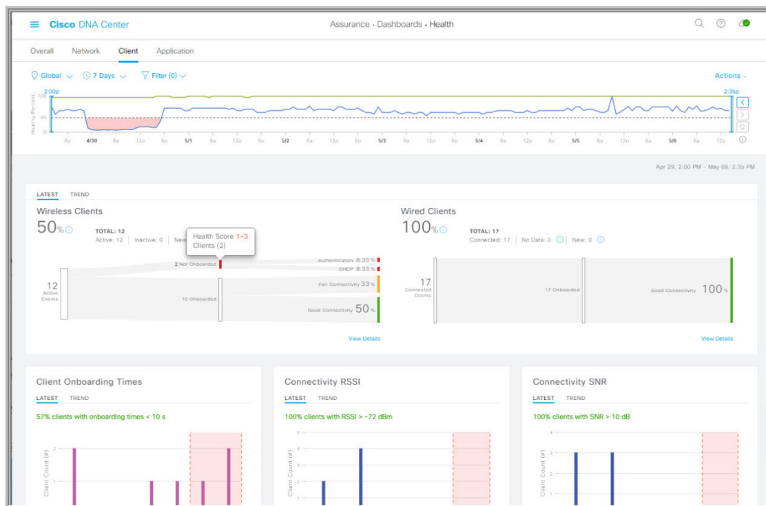
図 1: クライアントの正常性ダッシュボード
