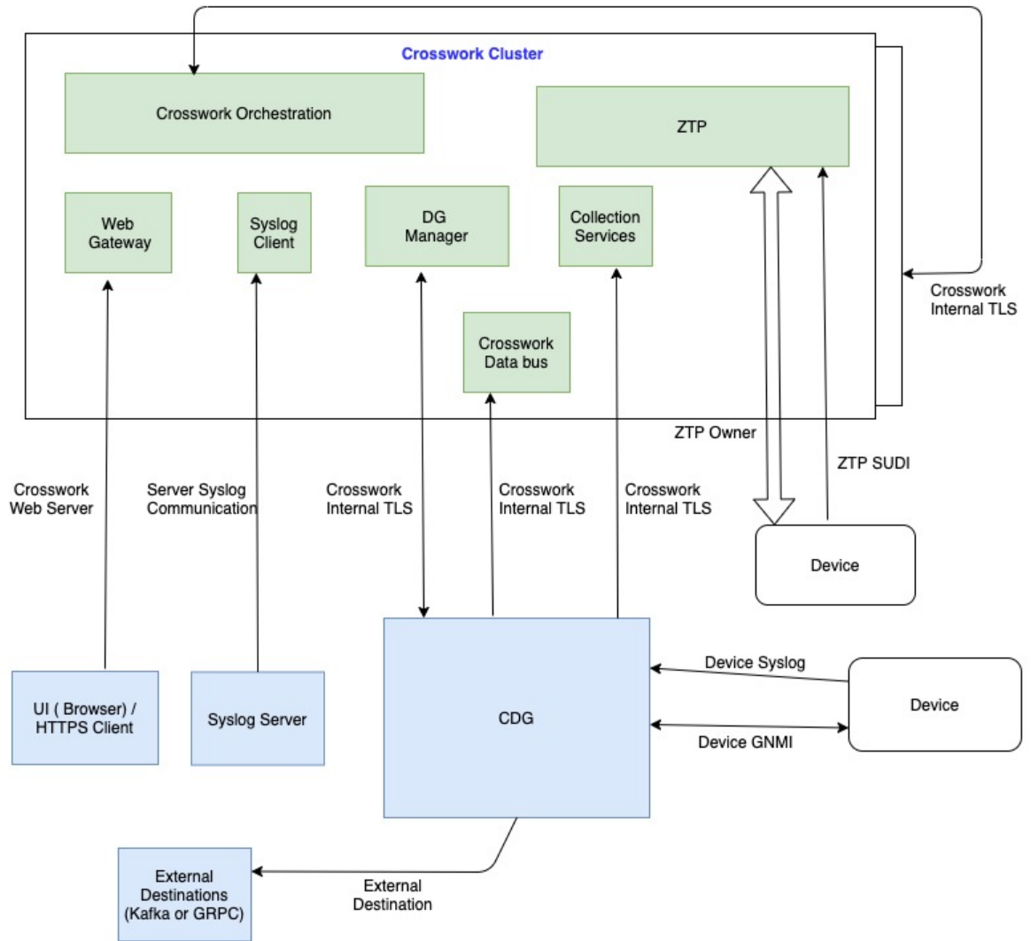
図 106: Cisco Crosswork の証明書
