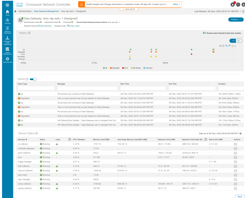
図 19: [データゲートウェイ (Data Gateway)] ウィンドウ
