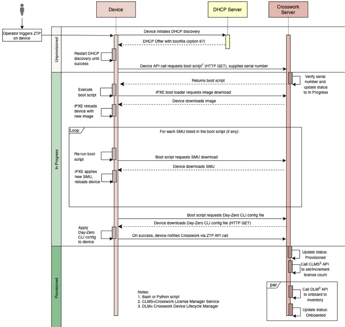
図 71:クラシック ZTP の処理
