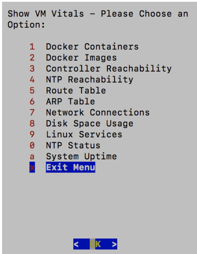
図 124: [VMのバイタルの表示 (Show VM Vitals) ]メニュー
