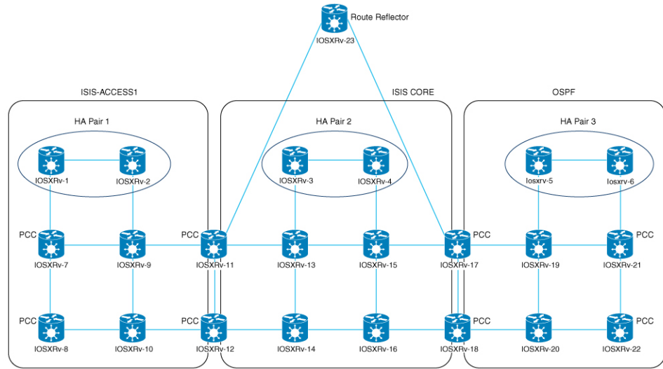
図 58: HA ペアが 3つの場合のトポロジの例
