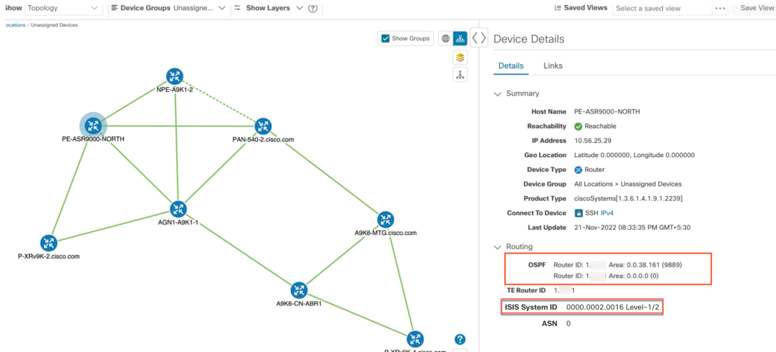
図 102: 複数の IGP : OSPF および ISIS プロセス
