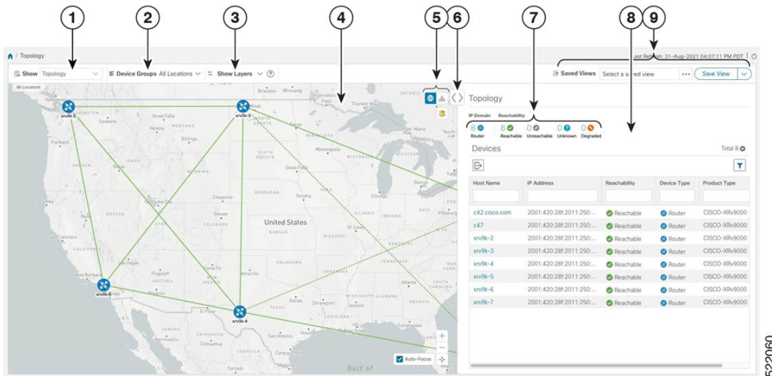
図 99 : Cisco Crosswork UI とトポロジマップ
