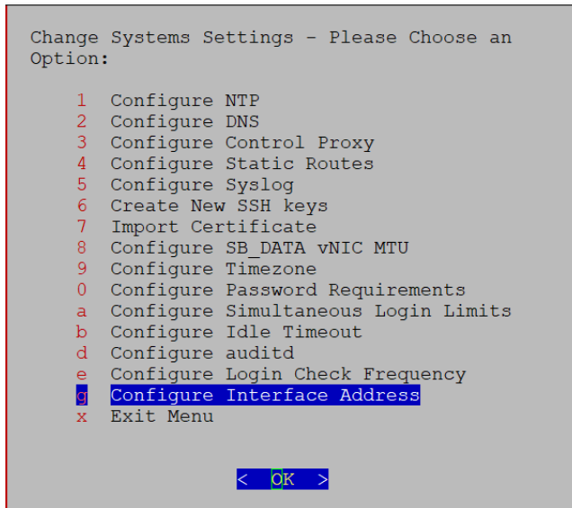
図 119: [システム設定の変更 (Change System Settings) ]メニュー
