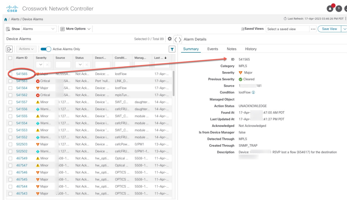
図 68: [アラームの詳細 (Alarm Details)] ウィンドウ: [概要 (Summary)] タブ
