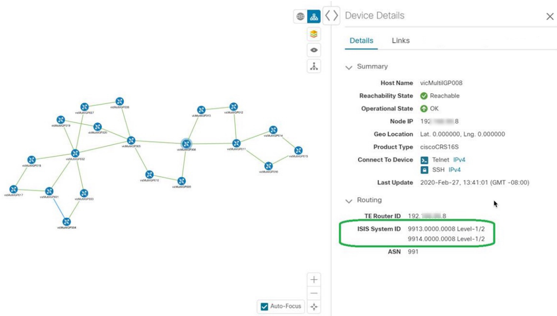
図 101: 複数の IGP : ISIS プロセス
