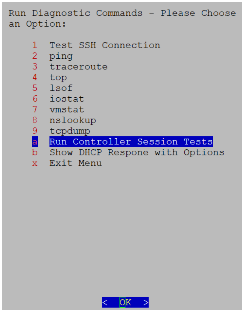
図 126: [コントローラセッションテストの実行 ( Run Controller Session Tests ) ]メニュー
