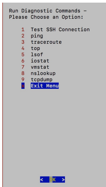
図 125: 診断の実行 (Run Diagnostics) ]メニュー
