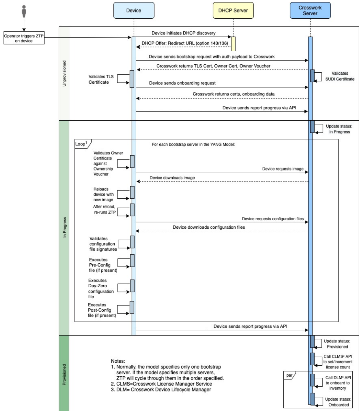
図 72:セキュア ZTP の処理
