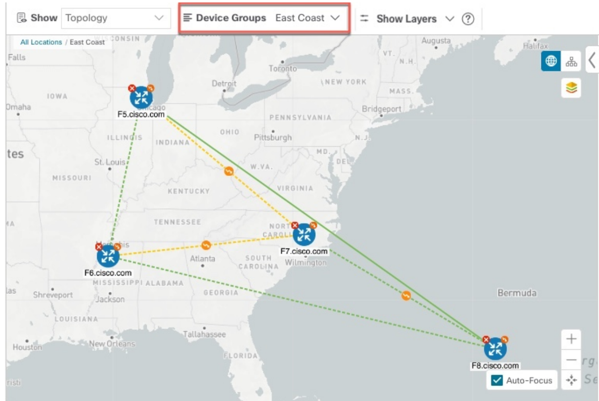
図 103: トポロジマップでのデバイスグループの選択
