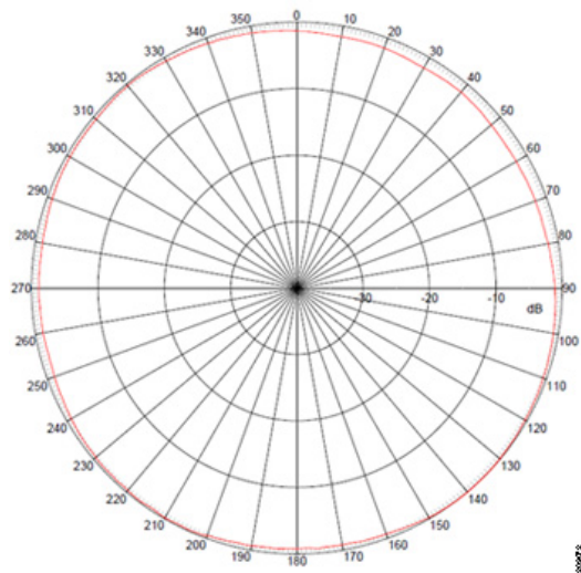
水平面内放射パターン (5 GHz)
