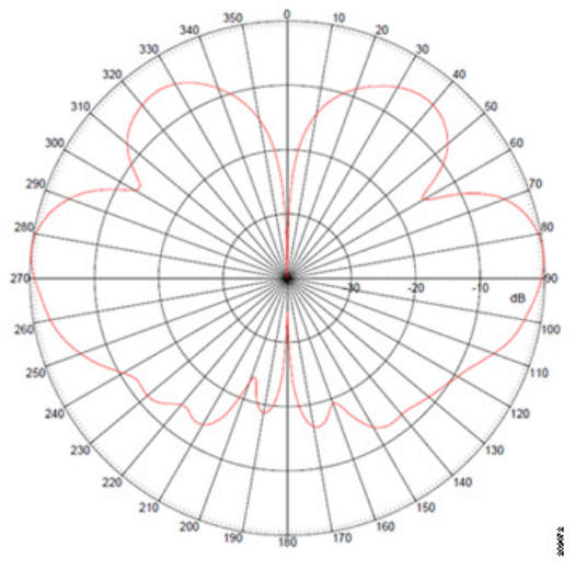
垂直面内放射パターン (5 GHz)
