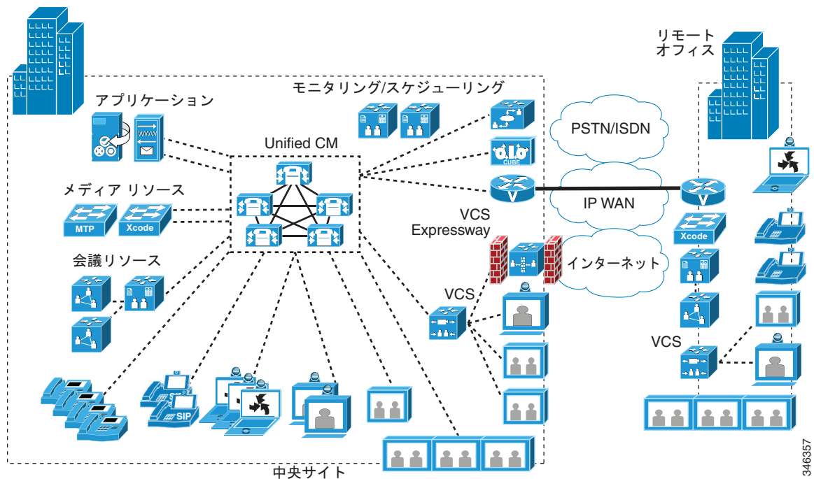
図 2-1 Cisco Unified Communications および Collaboration システムのアーキテクチャ
