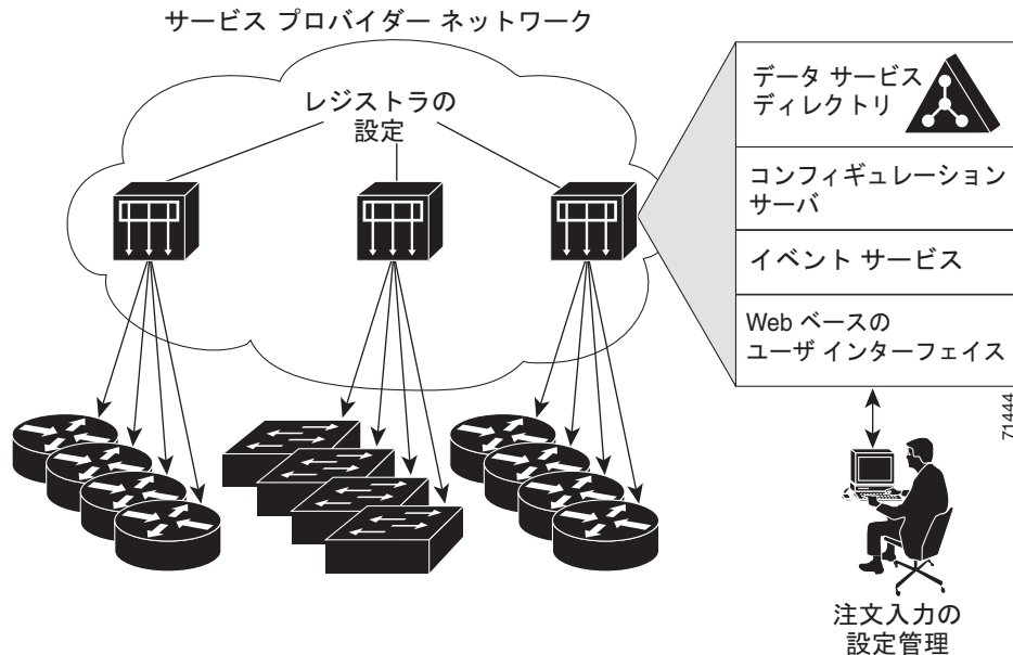
図 4-1 Configuration Registrar のアーキテクチャの概要
