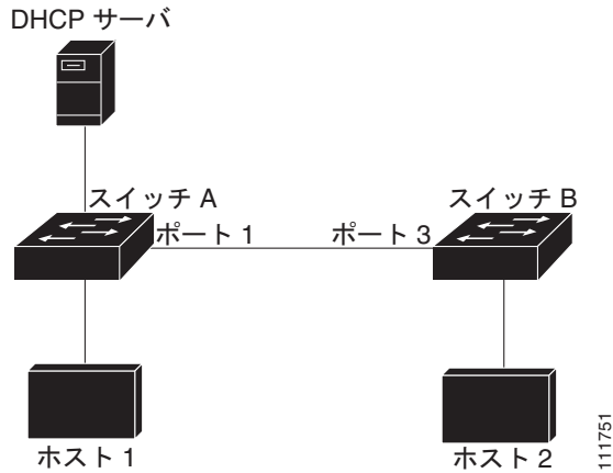
図 19-2 ダイナミック ARP インспекションのためにイネーブルにされた VLAN 上の ARP パケット検証
