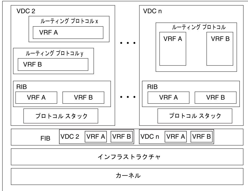
図 14-1 VDC 内の複数の VRF
