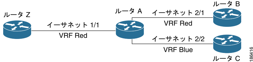
図 14-2 ネットワーク内の VRF
