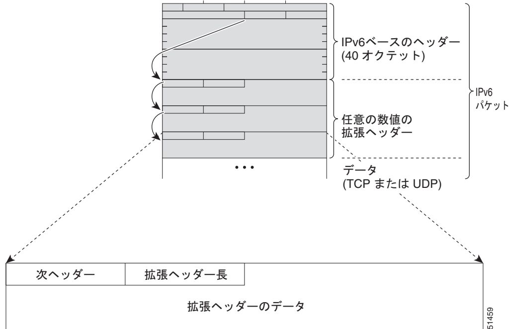
図 3-10 IPv6 拡張ヘッダーのフォーマット
