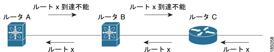
図 11-1 スプリット ホライズン ポイズン リバースを指定した RIP
