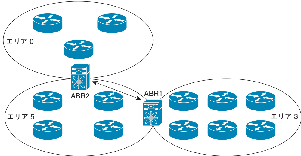
図 5-4 仮想リンク
