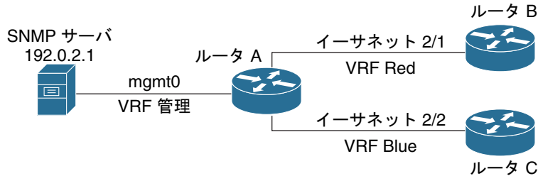
図 14-4 サービス VRF の到達可能性とフィルタリング
