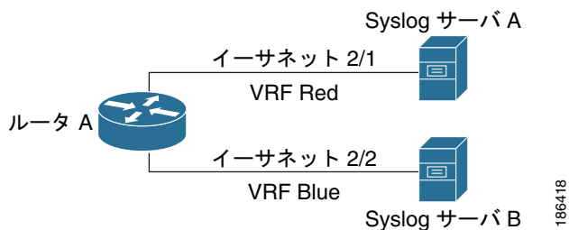
図 14-3 サービス VRF のフィルタリング
