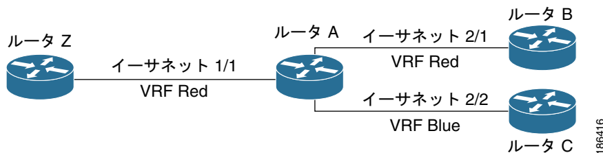
図 14-1 ネットワーク内の VRF
