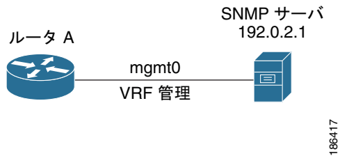
図 14-2 サービス VRF の到達可能性
