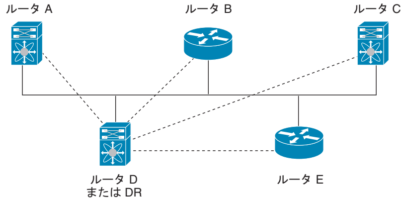
図 5-1 マルチアクセス ネットワークの DR
