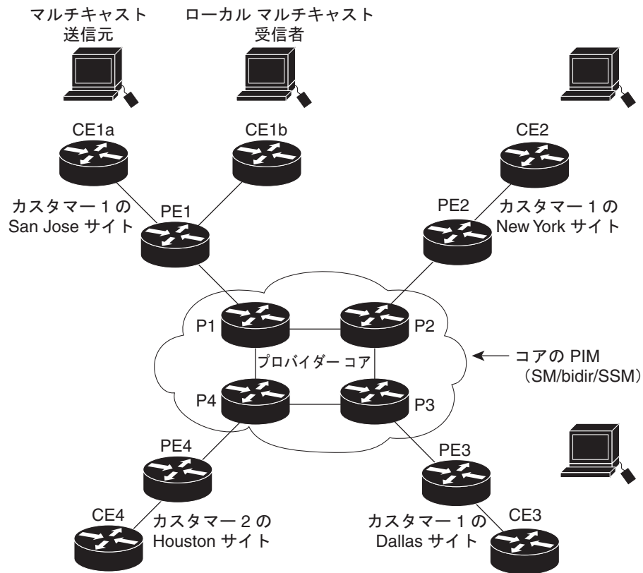
図 45-1 デフォルト マルチキャスト配信ツリーの概要
