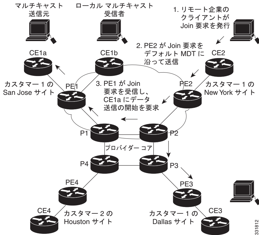
図 45-2 データ MDT の初期化
