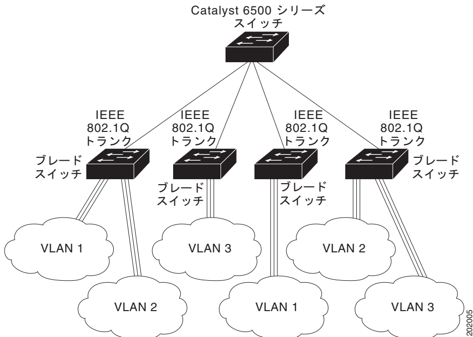
図 13-2 IEEE 802.1Q トランキング環境のスイッチ
