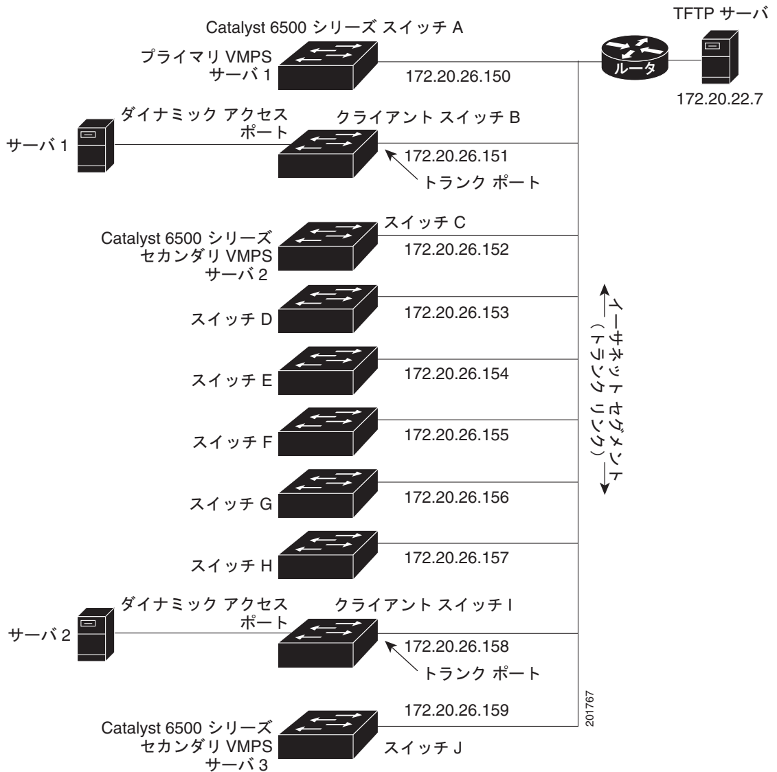
図 13-5 ダイナミック ポート VLAN メンバーシップの構成例
