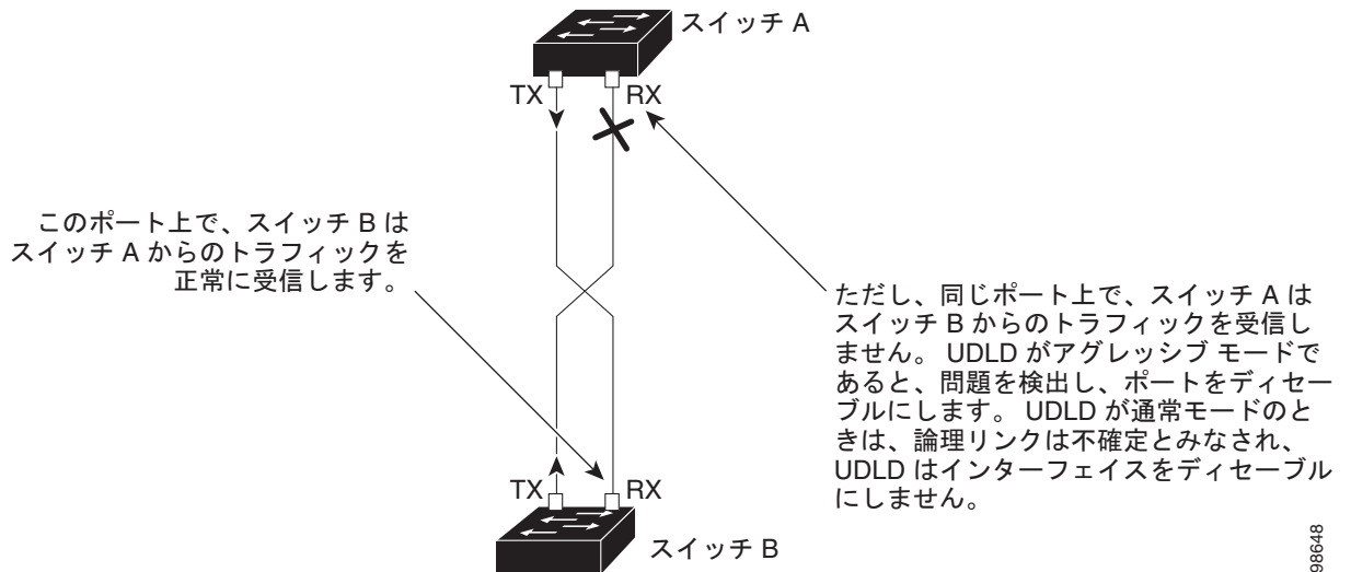
図 29-1 UDLD による単一方向リンクの検出
