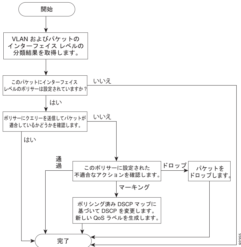
図 37-5 SVI のポリシー マップおよびマーキング フローチャート
