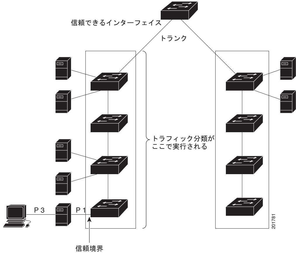
図 37-11 QoS ドメイン内のポートの信頼状態
