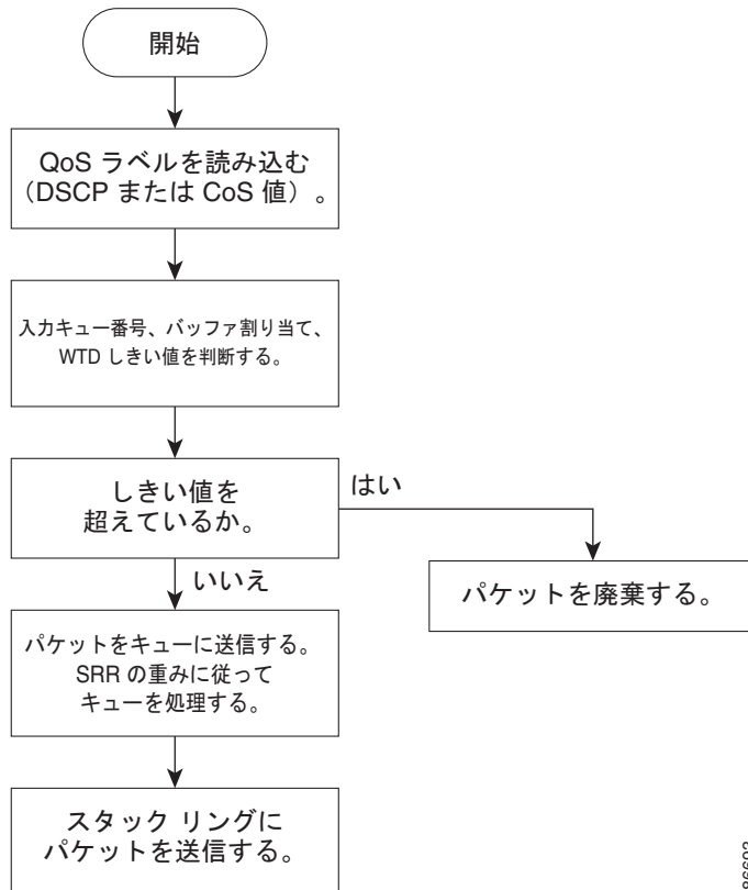
図 37-8 入力ポートのキューイングおよびスケジューリング フローチャート
