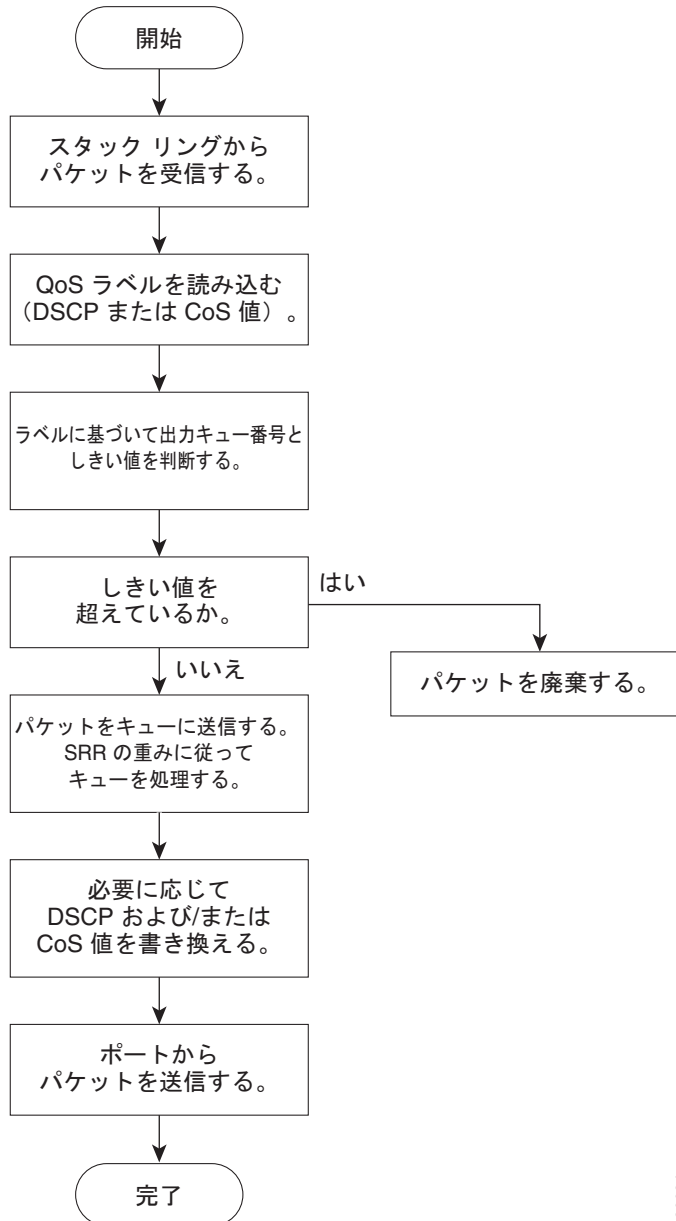
図 37-9 出力ポートのキューイングおよびスケジューリング フローチャート
