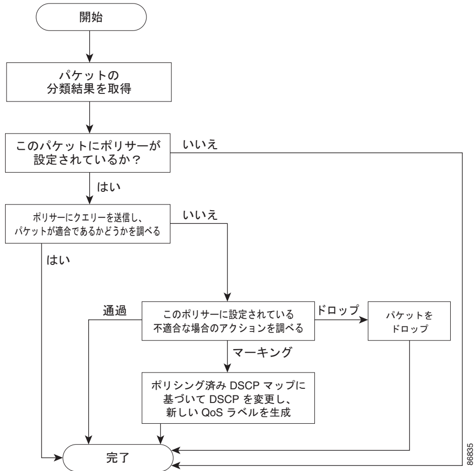
図 37-4 物理ポートのポリシングおよびマーキング フローチャート
