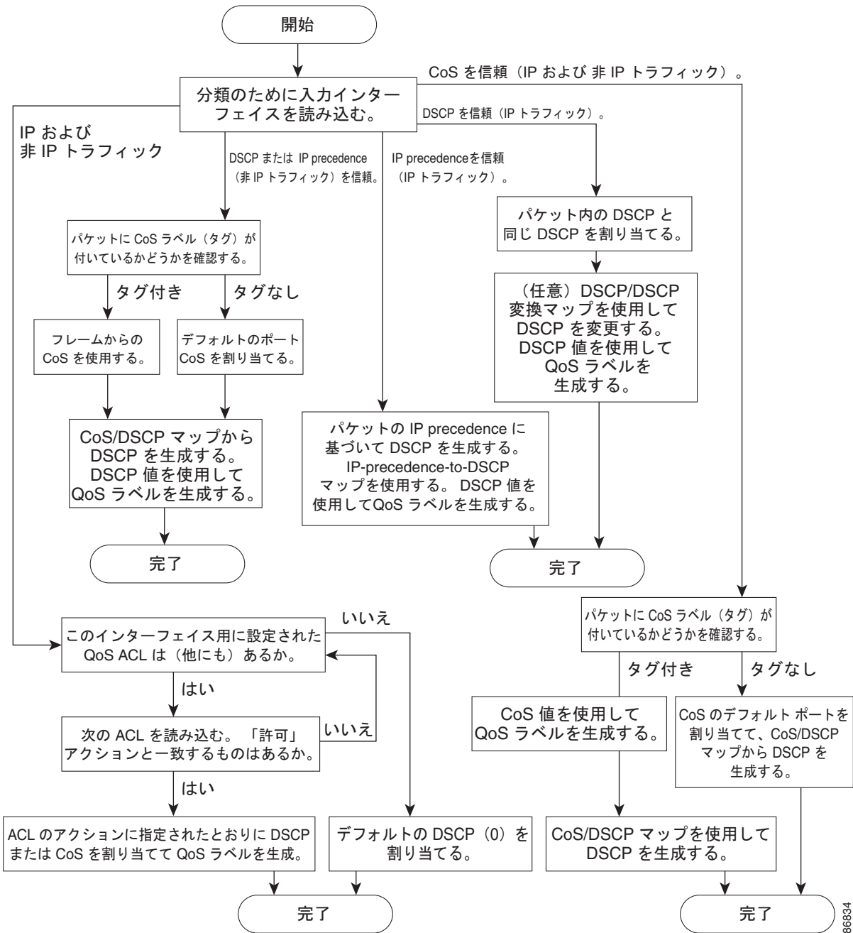
図 37-3 分類フローチャート
