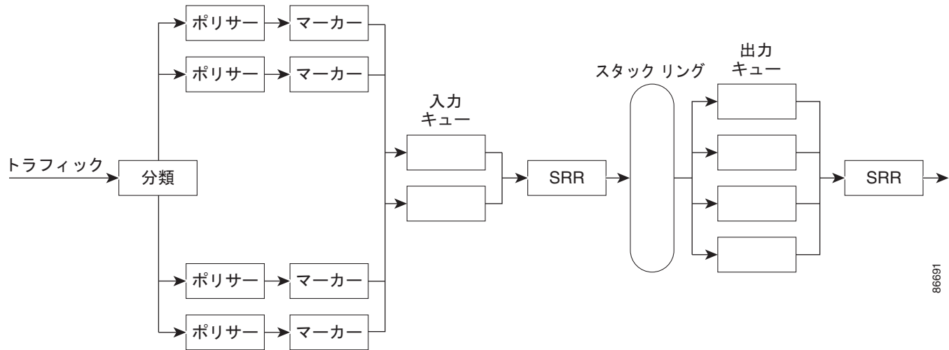
図 37-6 入力および出力キューの位置
