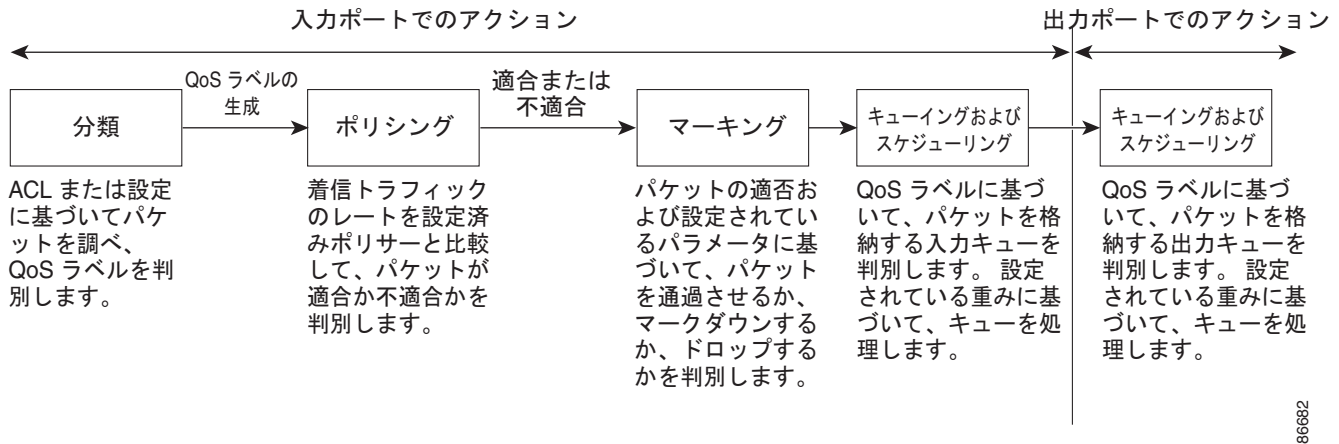
図 37-2 QoS の基本モデル
