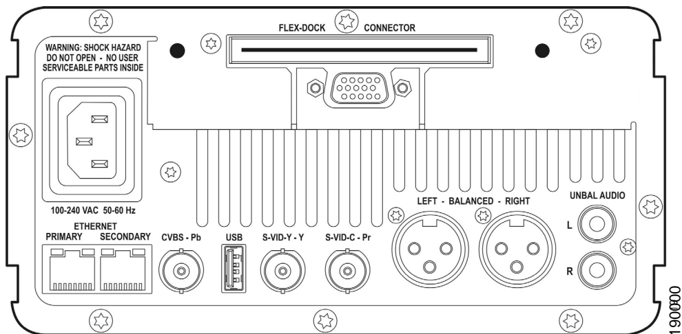
図 2 背面パネル
