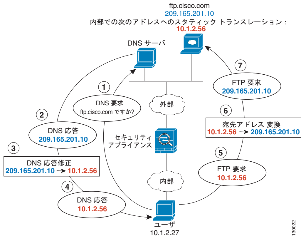
図 4-6 外部 NAT を使用する DNS 応答修正
