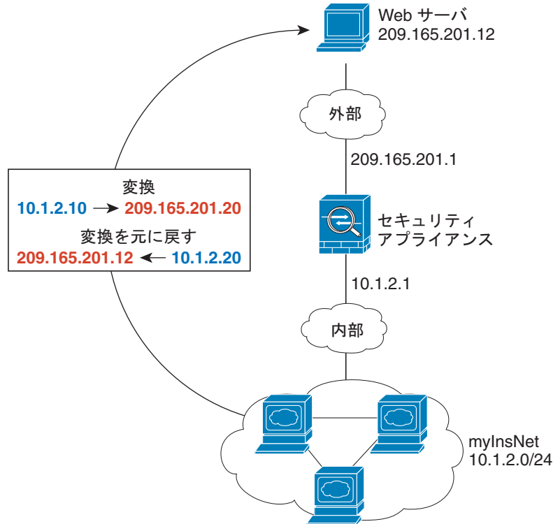
図 4-2 内部のダイナミック NAT、外部 Web サーバのスタティック NAT
