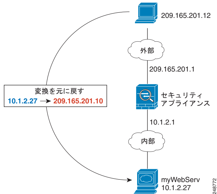
図 4-1 内部 Web サーバのスタティック NAT
