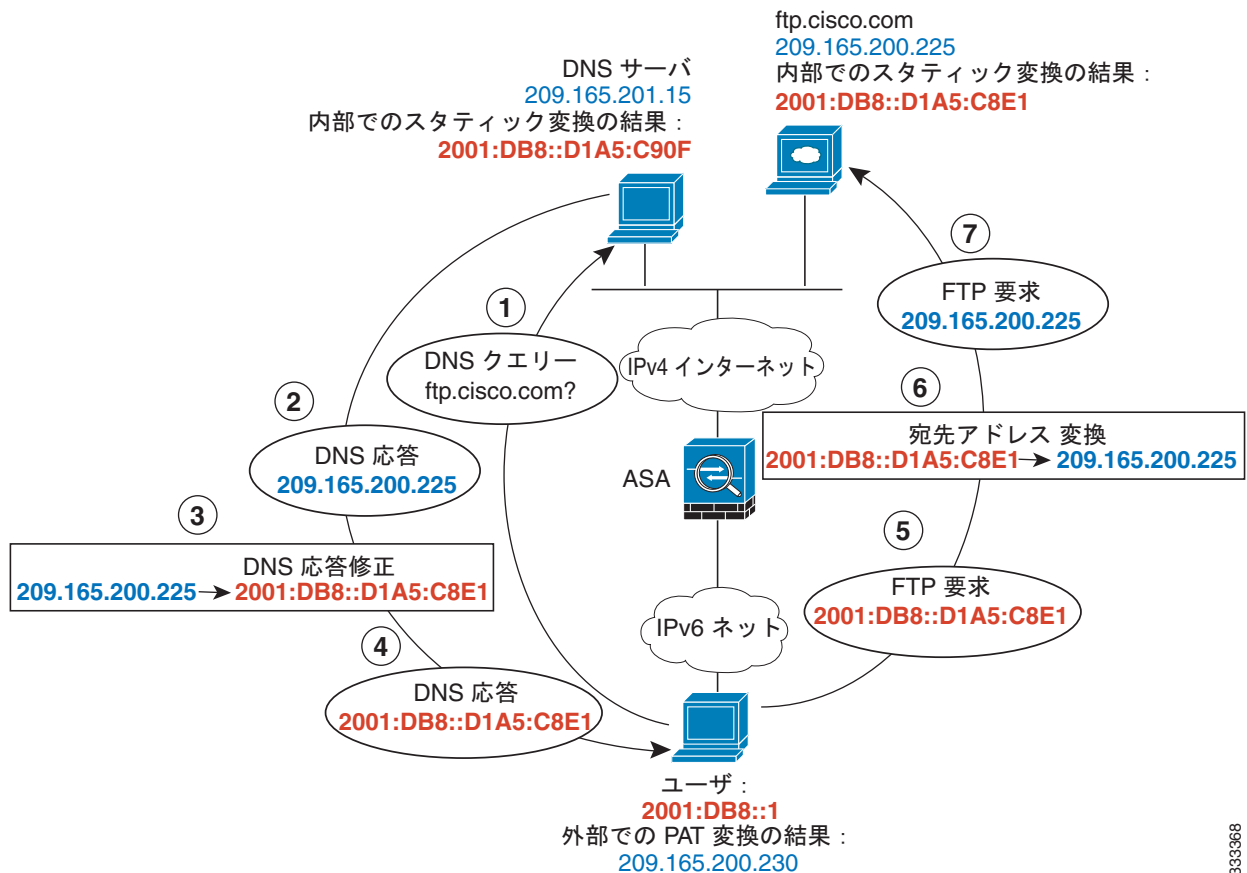
図 4-7 外部 NAT を使用する DNS 応答修正
