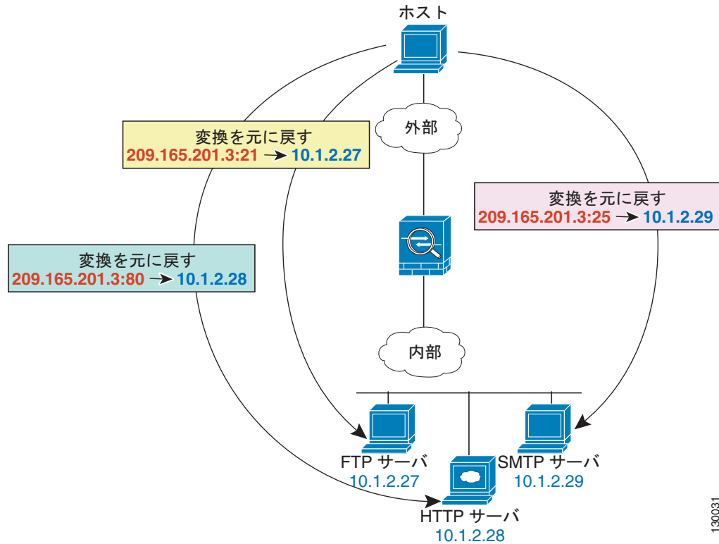
図 4-4 ポート変換を設定したスタティック NAT
