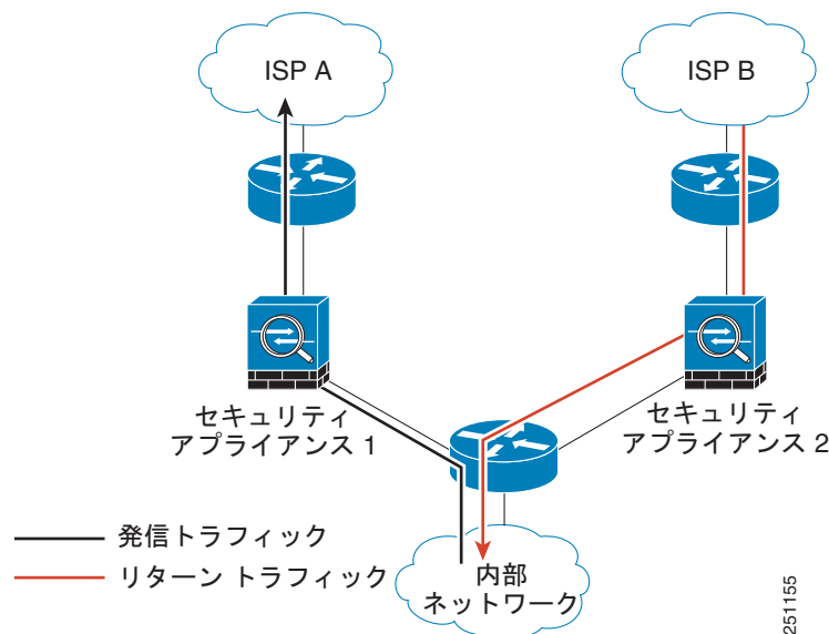
図 19-1 非対称ルーティング
