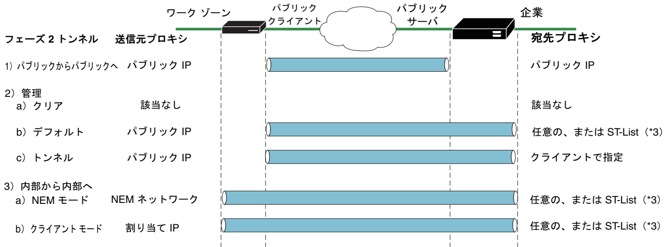
図 75-1 Cisco ASA 5505 用の Easy VPN ハードウェア クライアント トンネリング オプション
