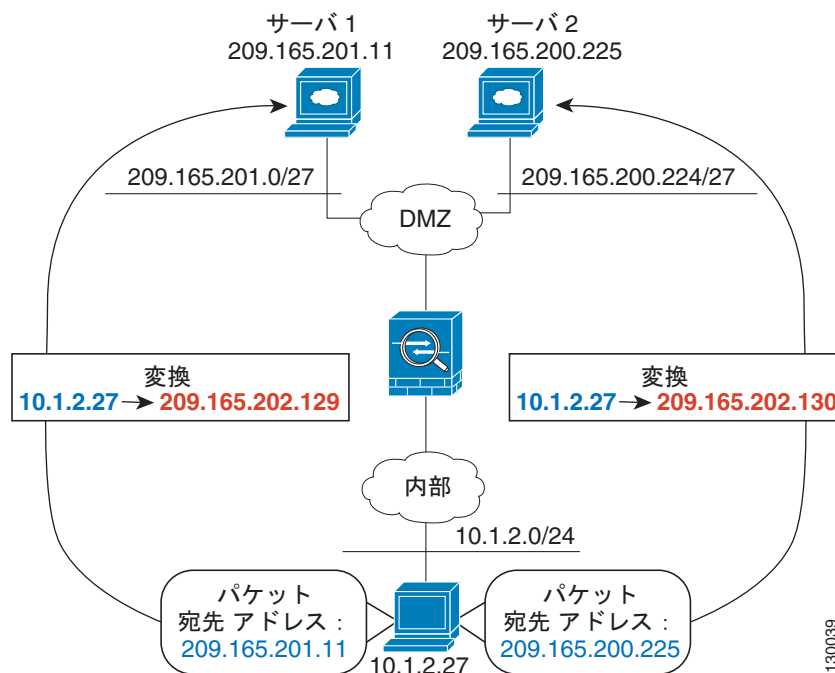
図 35-1 異なる宛先アドレスを使用する Twice NAT
