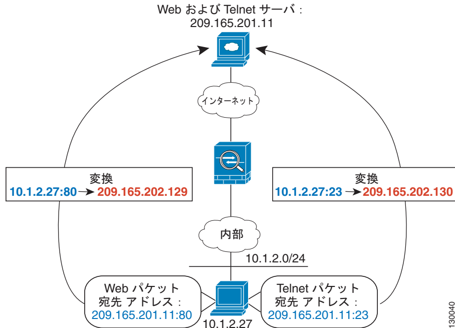
図 35-2 異なる宛先ポートを使用する Twice NAT
