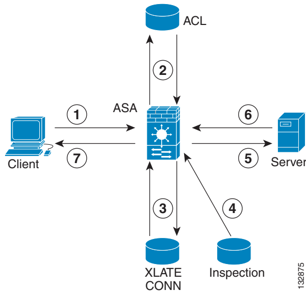
図 46-1 インспекション エンジンの動作
