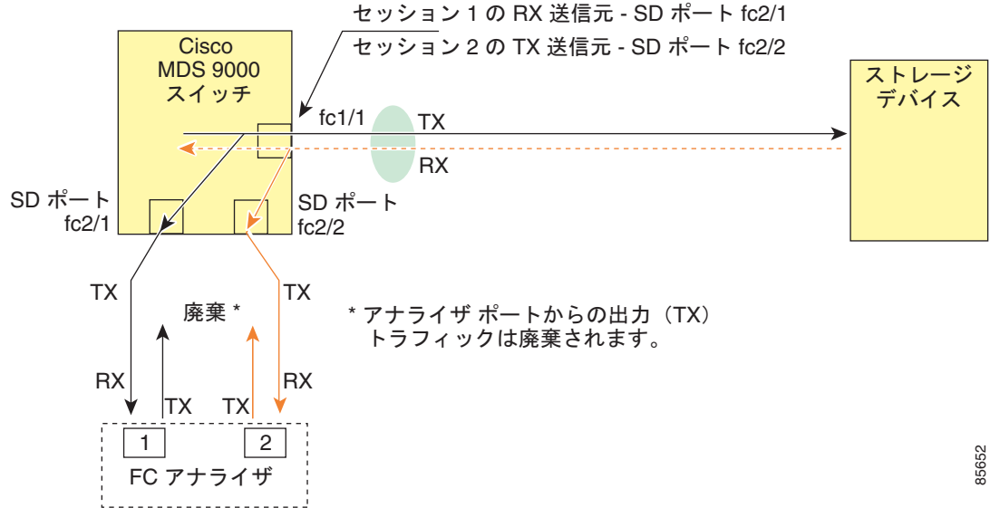
図 62-9 SPAN を使用した場合のファイバチャネル アナライザの使用方法
