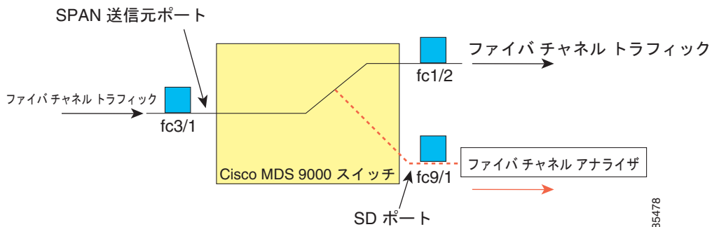
図 62-1 SPAN の送信
