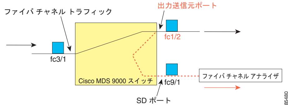
図 62-3 出力方向からの SPAN トラフィック
