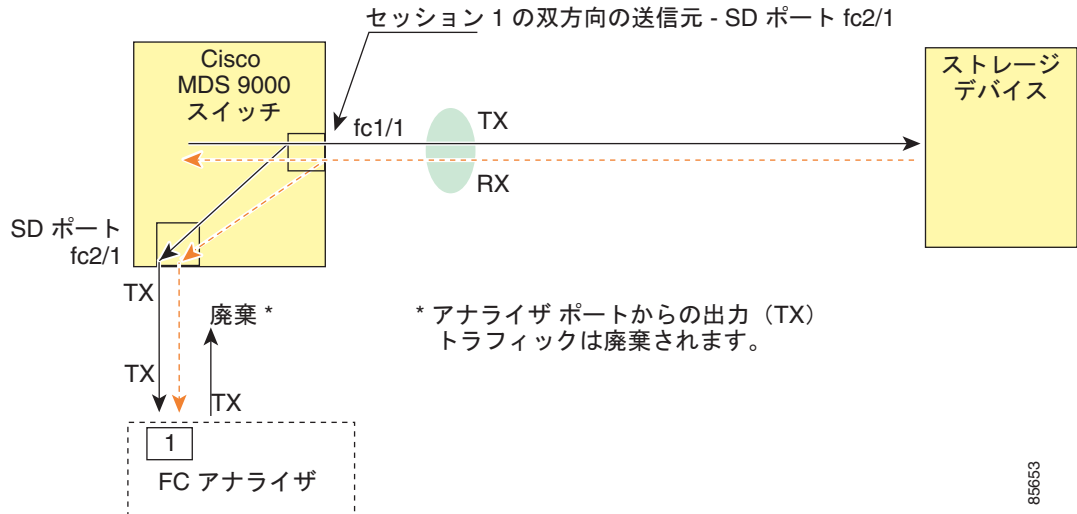
図 62-10 単一 SD ポートを使用した場合のファイバ チャンネル アナライザ
