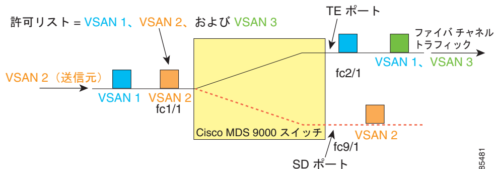
図 62-4 送信元としての VSAN
