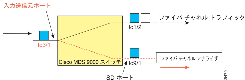
図 62-2 入力方向からの SPAN トラフィック
