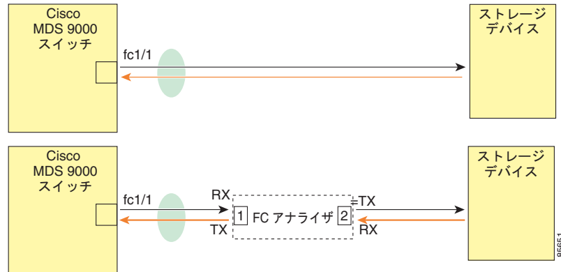
図 62-8 SPAN を使用しない場合のファイバチャネル アナライザの使用方法
