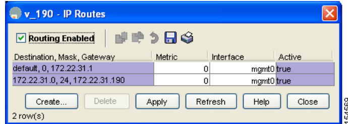
図 54-12 Device Manager の [IP Routing Configuration] ダイアログボックス
