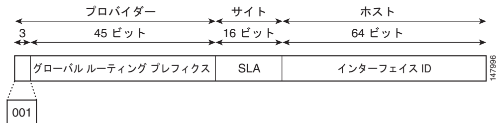
図 54-1 グローバルアドレスの形式
