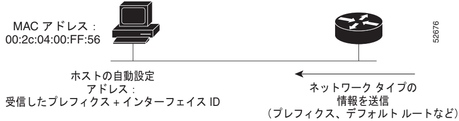
図 54-8 IPv6 ステートレス自動設定
