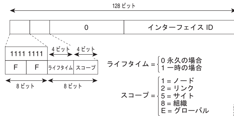
図 54-4 IPv6 マルチキャストアドレスの形式
