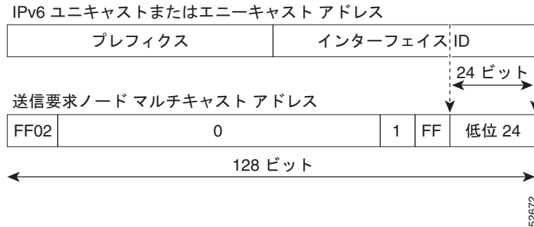
図 54-5 IPv6 送信要求ノード マルチキャスト アドレスの形式
