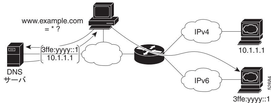
図 54-10 デュアル IPv4 および IPv6 プロトコル スタック アプリケーション
