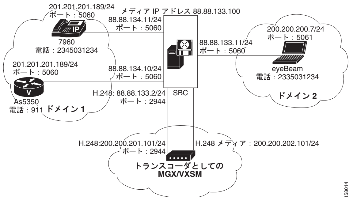
図 A-1 Cisco XR 12000 シリーズ ルータ上の SBC のトポロジ
