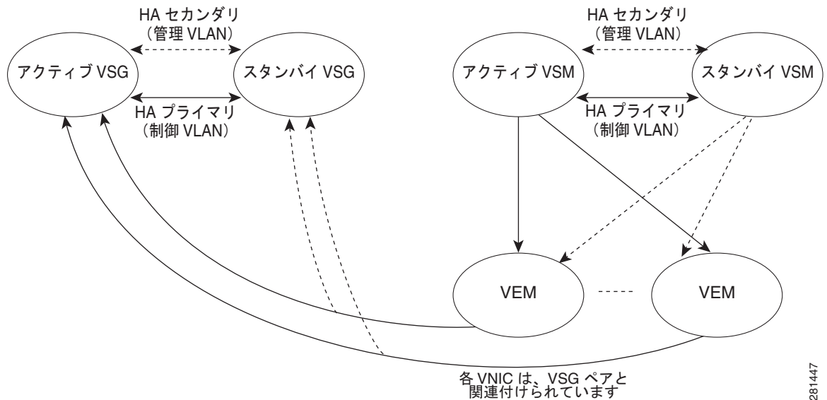
図 6-1 Cisco VSG のハイ アベイラビリティ
