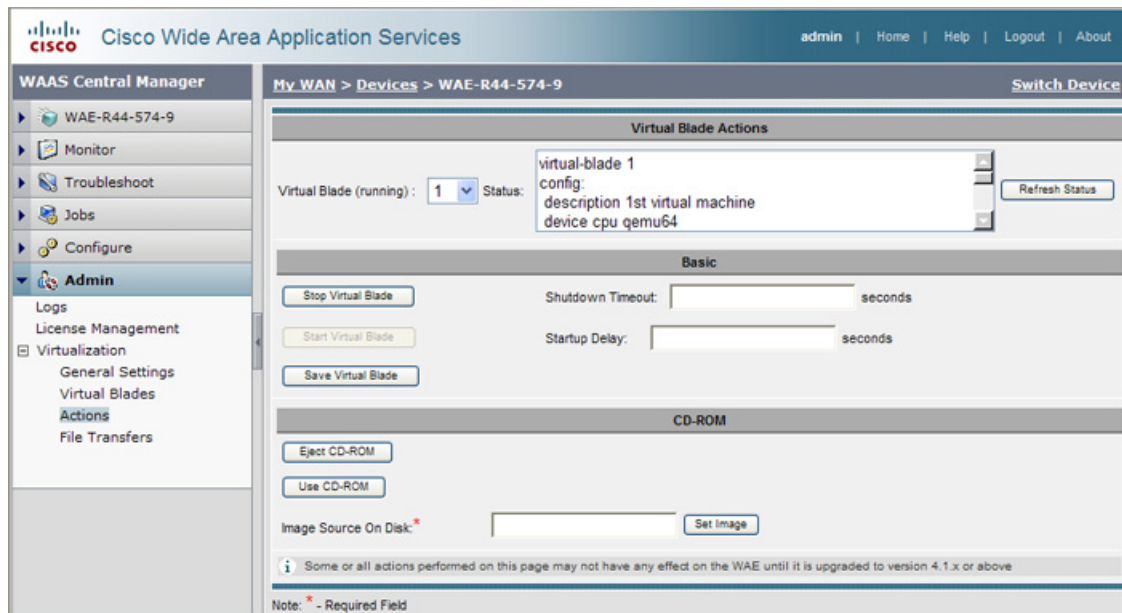
図 13-3 [Virtual Blade Actions] ウィンドウ
