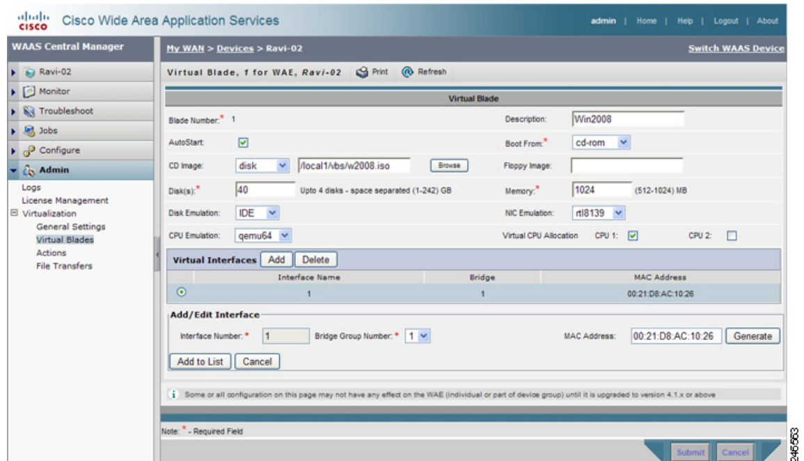
図 13-2 [Virtual Blade Configuration] ウィンドウ
