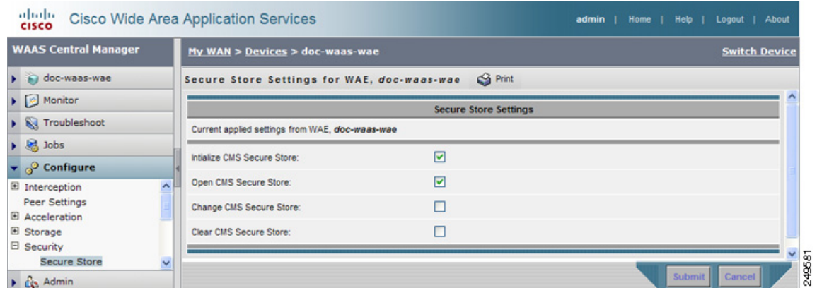
図 9-1 [Secure Store Settings] ウィンドウ
