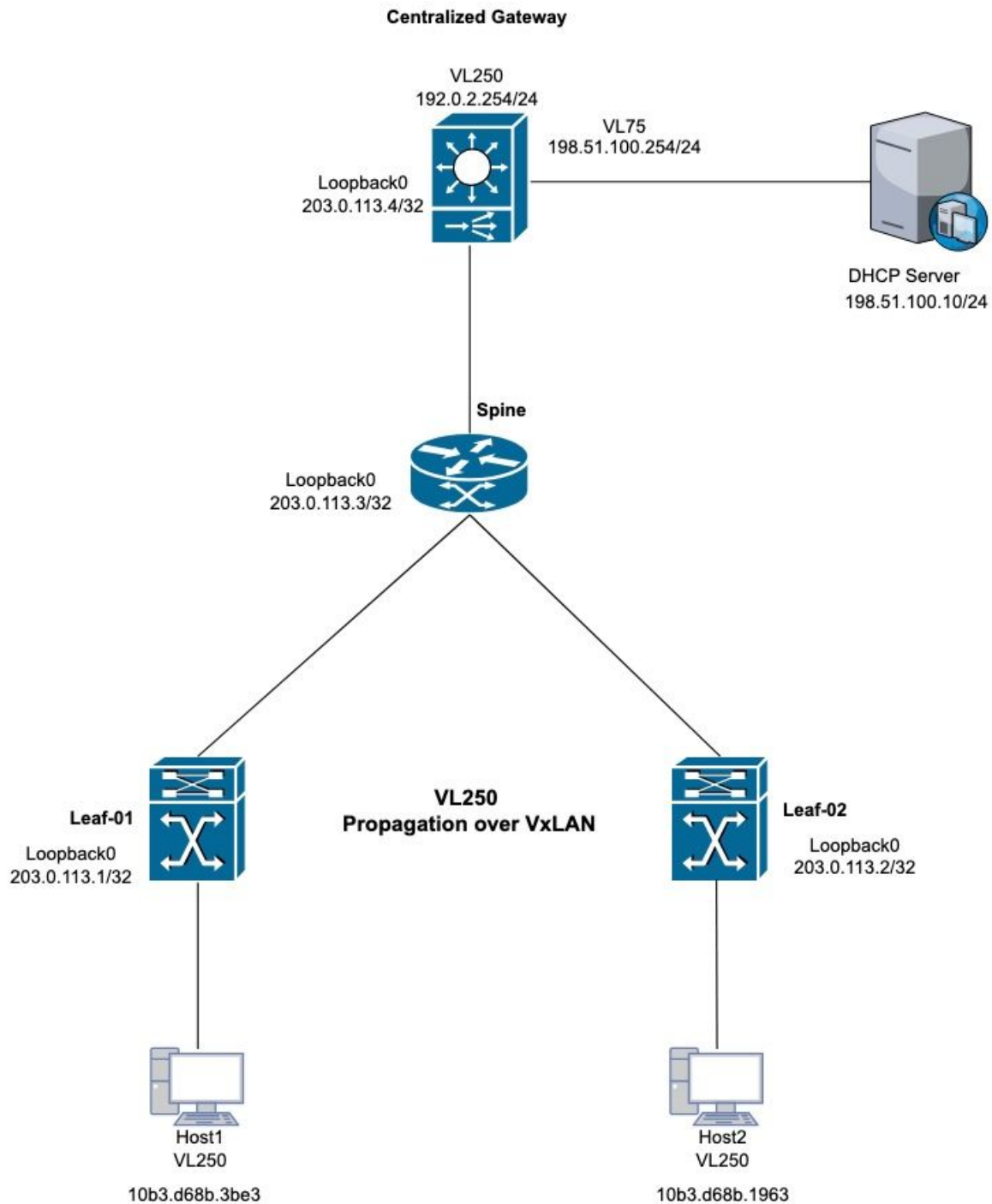
DHCP VxLAN拓撲
