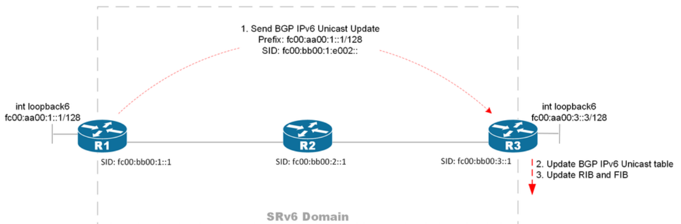
圖2.啟用封裝srsv6後的BGP信令流
