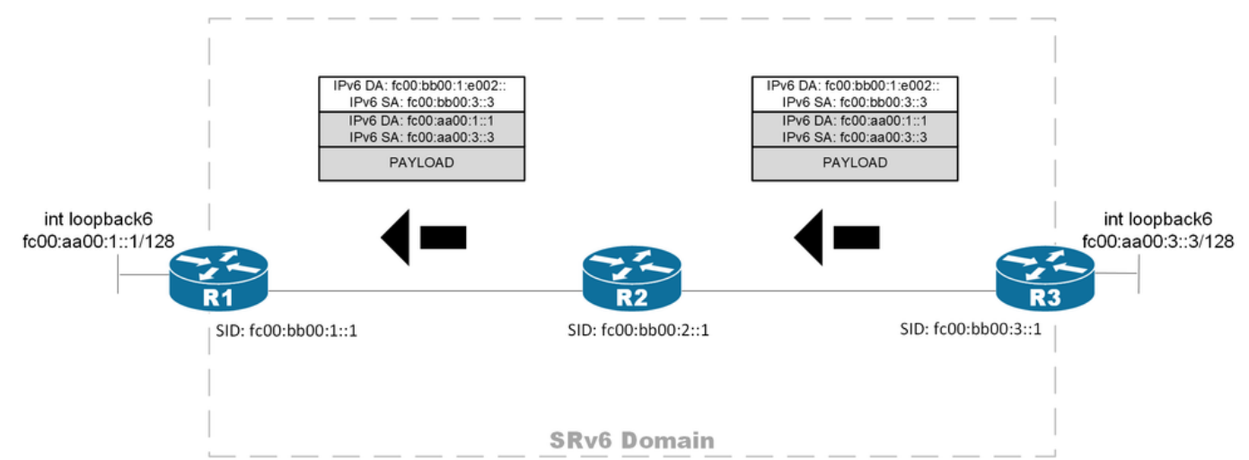
圖4.通過SRv6的BGP IPv6單播路徑上的資料包處理
