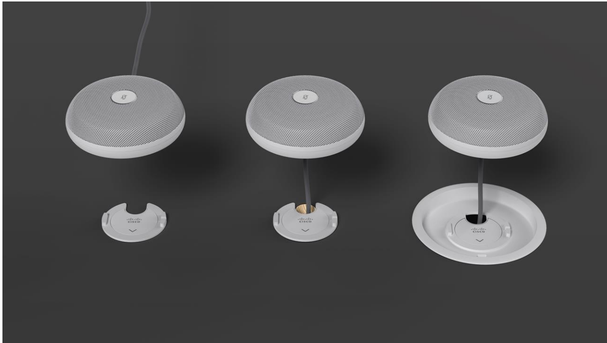
圖 3. Table Microphone Pro 的安裝選項。
