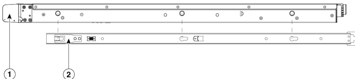
图 1: 将内滑轨固定到机箱的侧面
