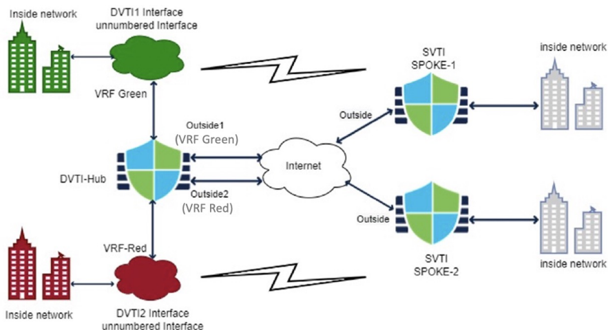
图 2: 具有多个虚拟路由器和动态 VTI 的站点间 VPN
