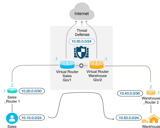
图 1: 互联两个虚拟路由器 - 示例
