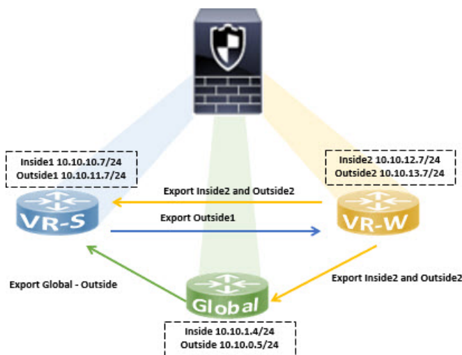
图 3. 使用 BGP 设置来互连虚拟路由器
