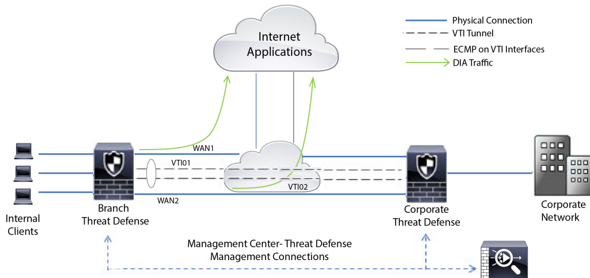
图 1: 在 防火墙管理中心 中的分支机构 上配置策略型路由
