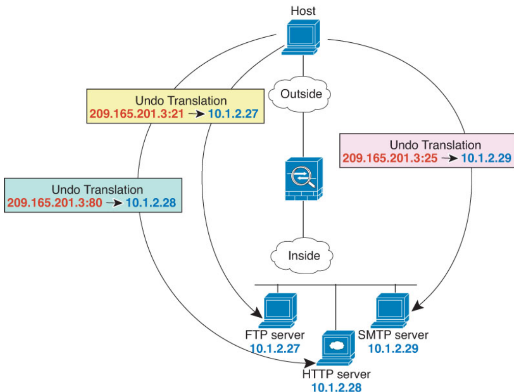
图 18: 支持端口转换的静态 NAT
