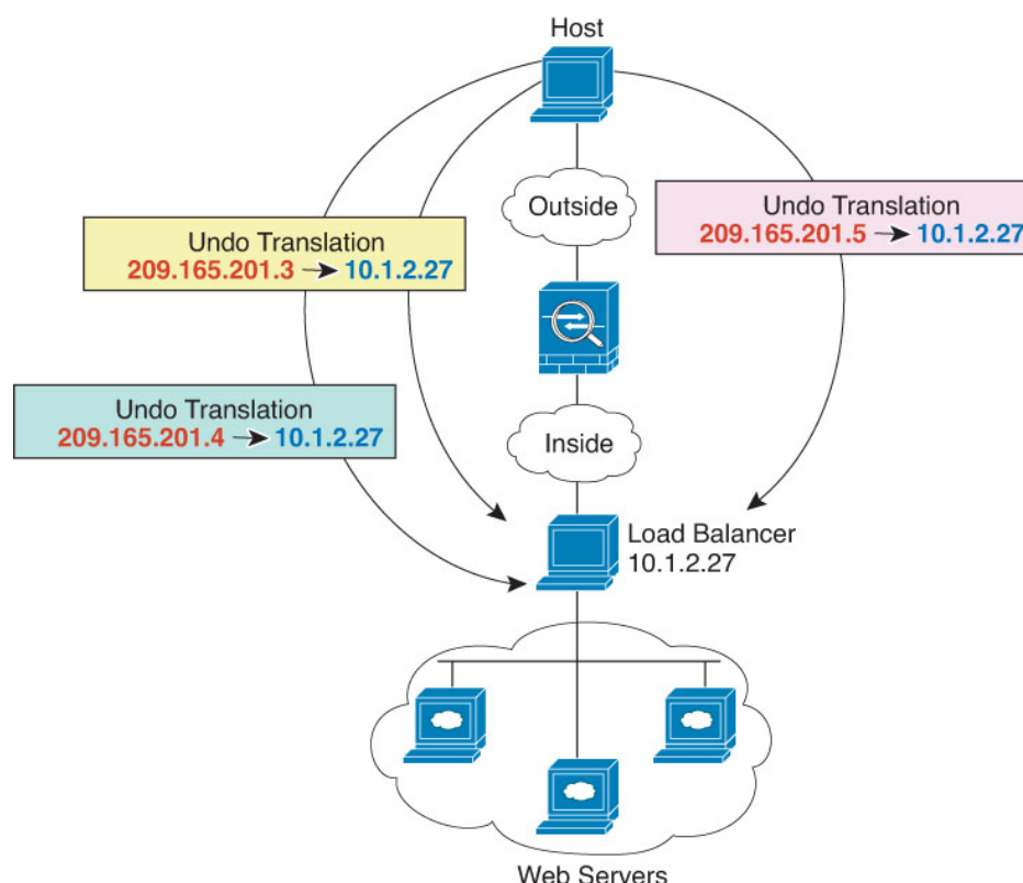
图 17: 内部负载均衡器的一对多静态 NAT
