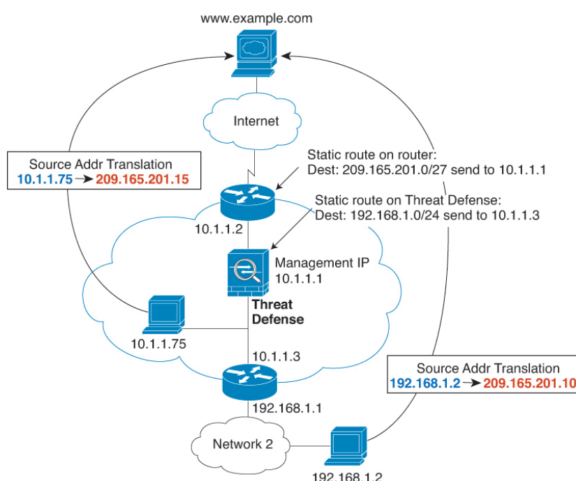
图 2: NAT 示例：透明模式
