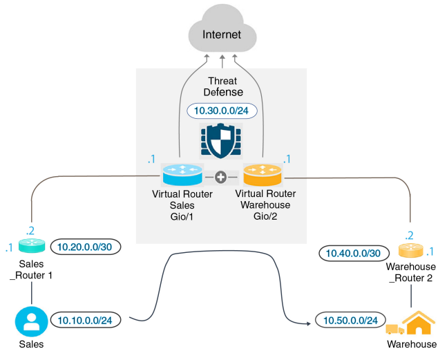
图 1: 互联两个虚拟路由器 - 示例
