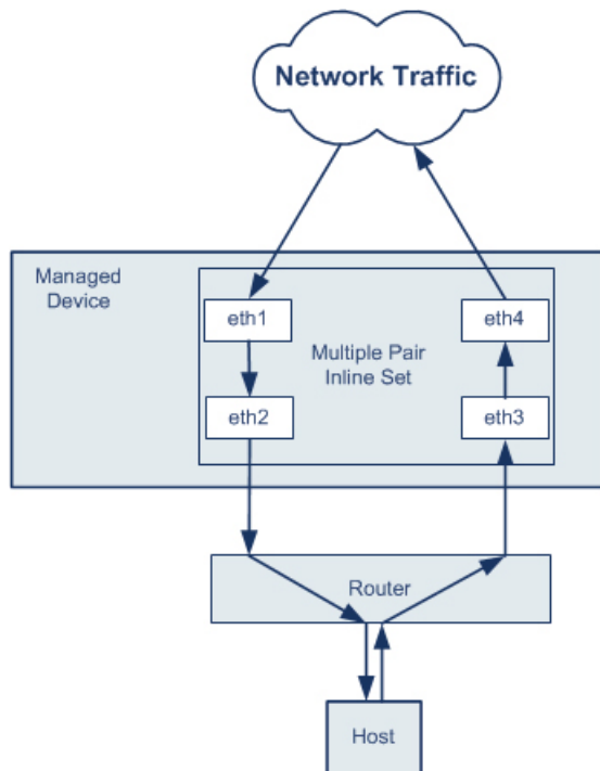
图 1: 异步路由
