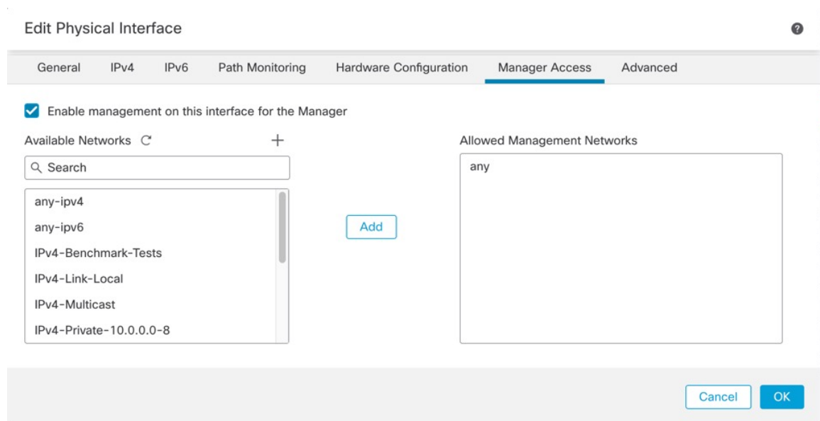
图 19: 管理器访问
