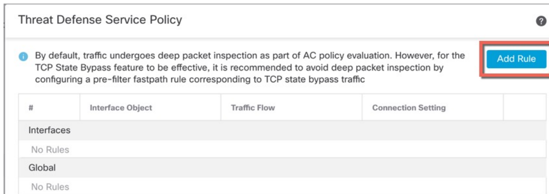
图 10: 添加规则
