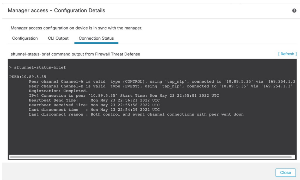
图 40: 连接状态
