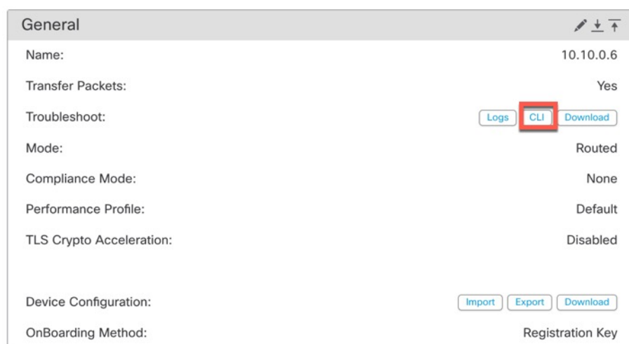
图 5: CLI
