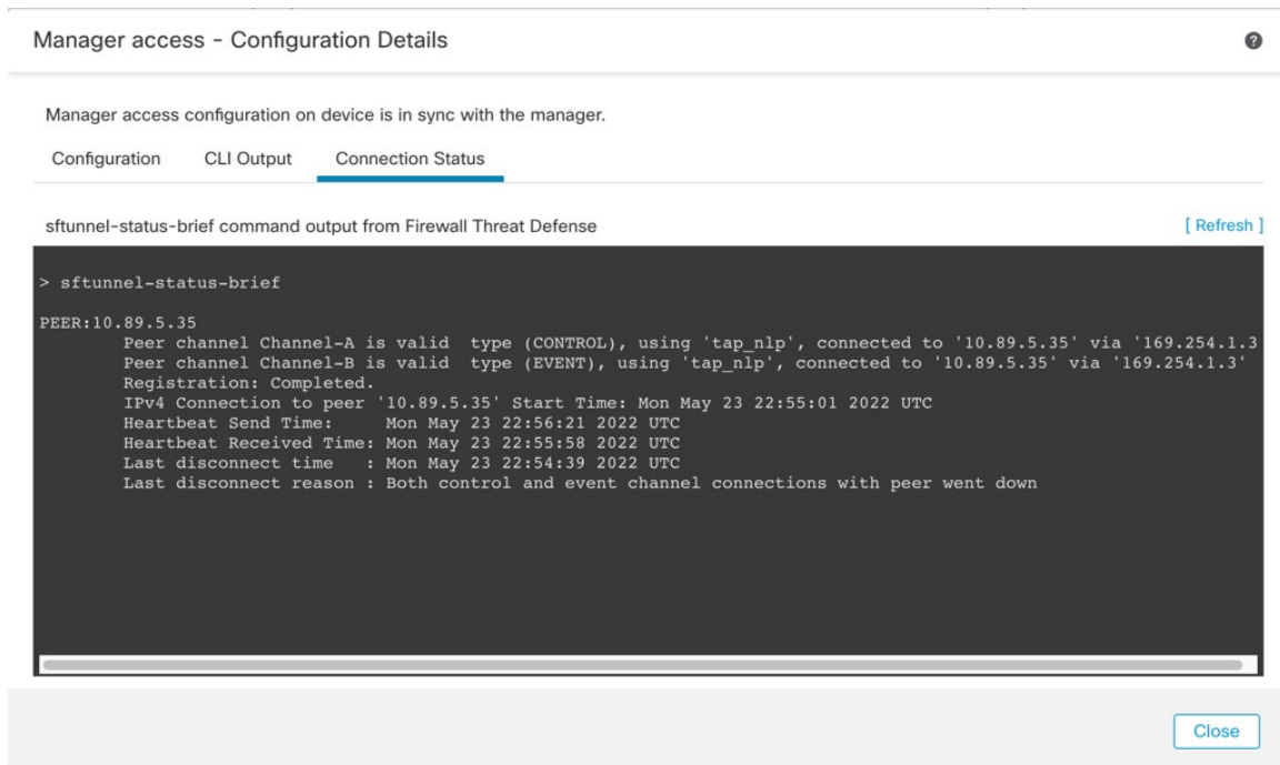
图 29: 连接状态
