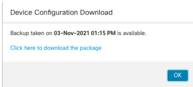
图 10: 下载软件包
