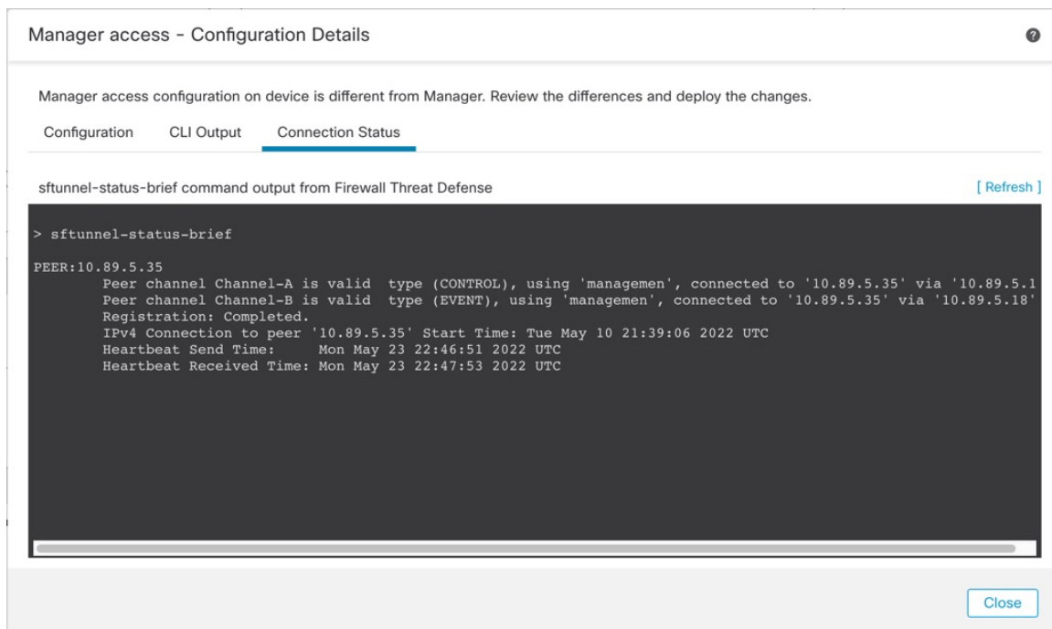
图 39: 连接状态
