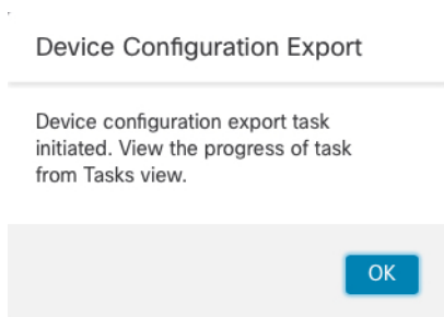
图 8: 确认导出
