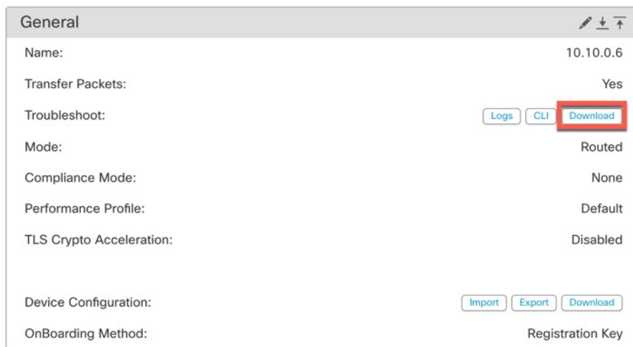
图 4: 下载
