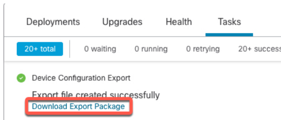
图 9: 导出任务
