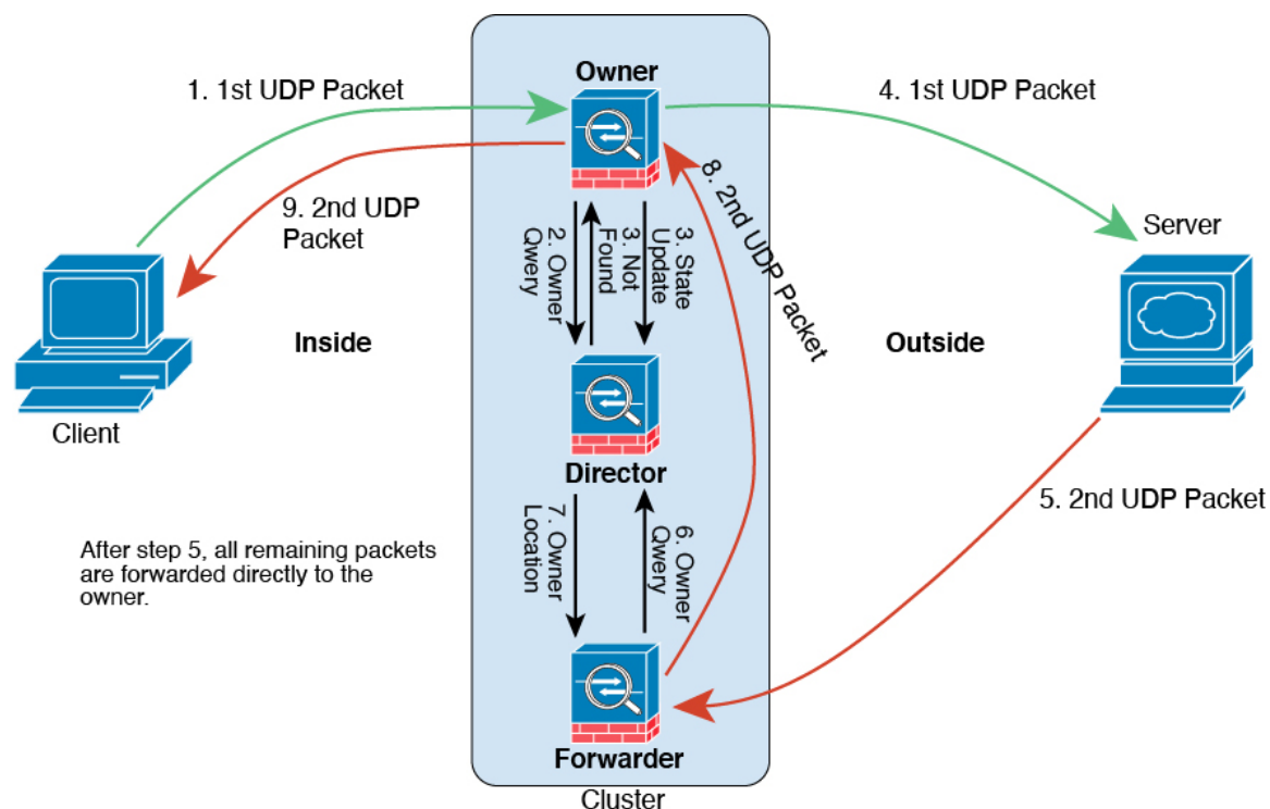
1. 图 37: ICMP 和 UDP 数据流
