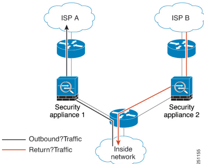
图 1: 非对称路由
