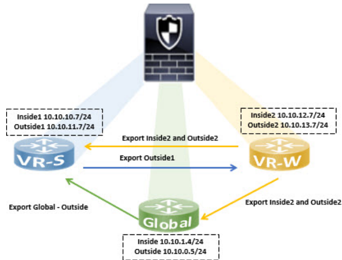
图 2: 使用 BGP 设置来互连虚拟路由器
