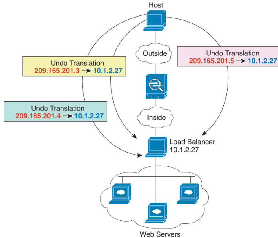
图 16: 内部负载均衡器的一对多静态 NAT
