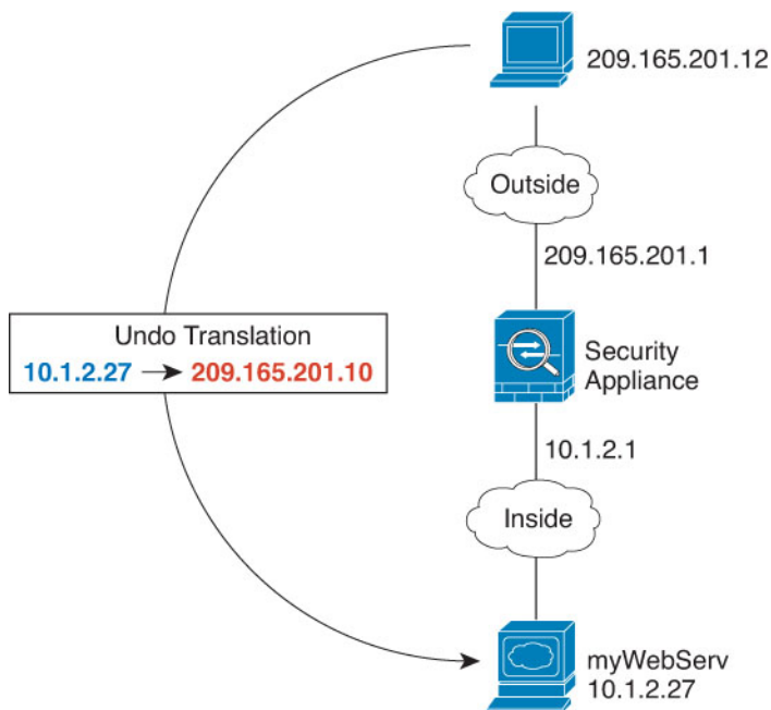
图 14: 面向内部 Web 服务器的静态 NAT
