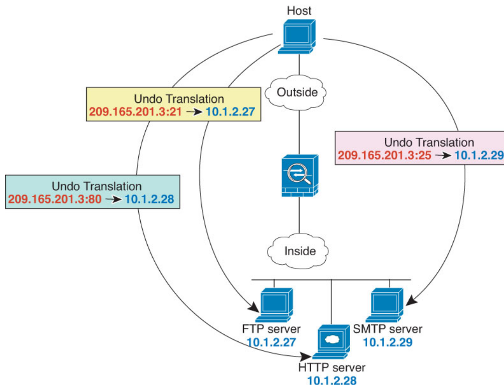
图 17: 支持端口转换的静态 NAT
