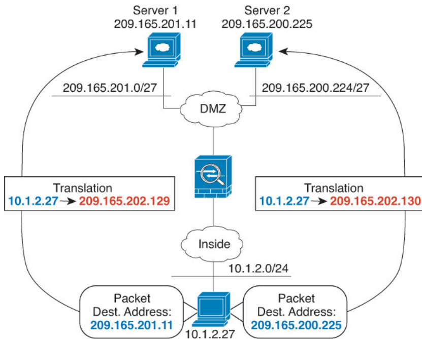
图 18: 具有不同目标地址的手动 NAT
