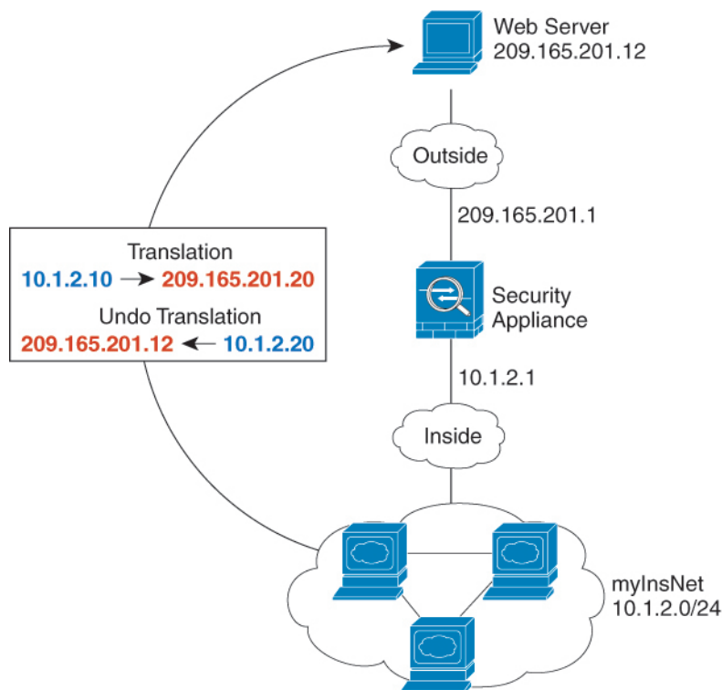
图 15: 面向内部 Web 服务器的动态 NAT, 面向外部 Web 服务器的静态 NAT
