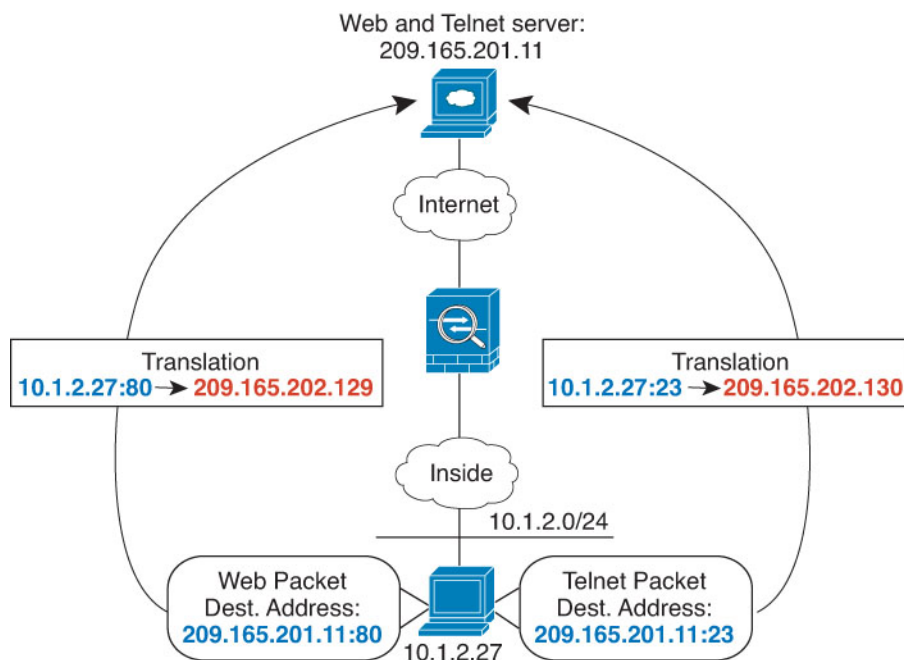
图 19: 具有不同目标端口的手动 NAT
