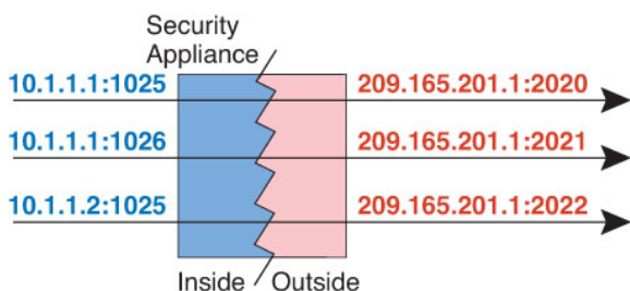
图 6: 动态 PAT
