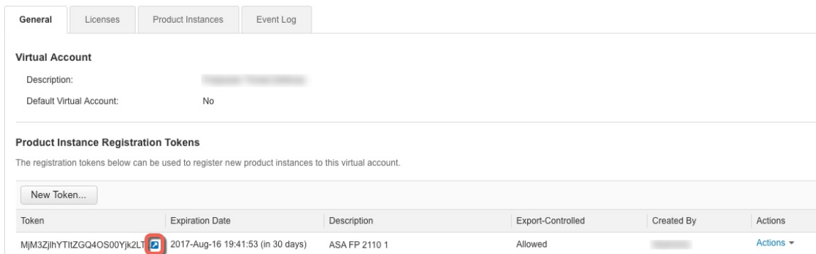
图 3: 复制令牌
