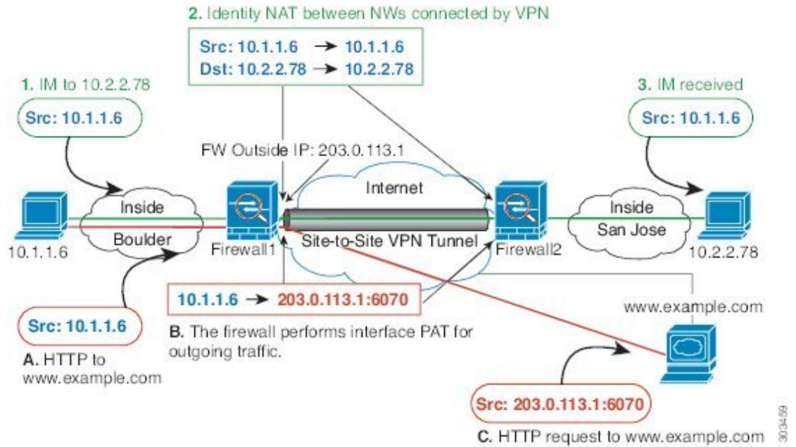
图 21: 用于站点间 VPN 的接口 PAT 和身份 NAT
