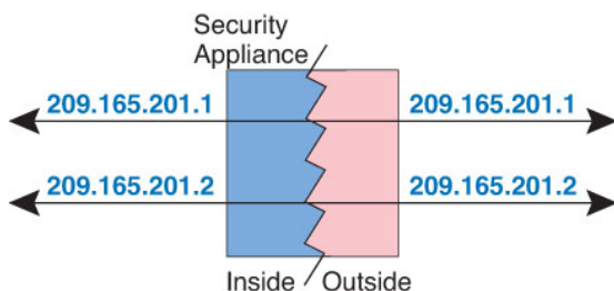
图 14: 身份 NAT
