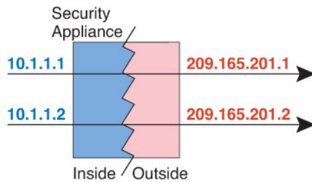
图 5: 动态 NAT
