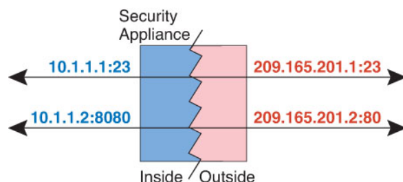
图 9: 支持端口转换的典型静态 NAT 场景
