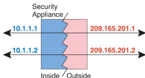
图 8: 静态 NAT
